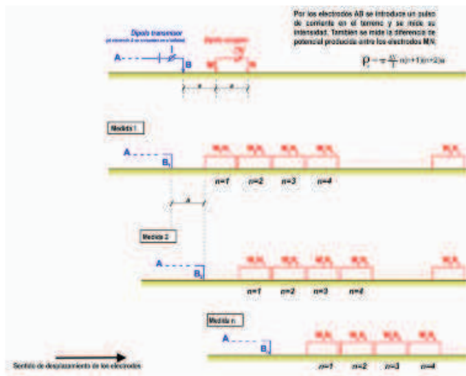
Figura 7. Dispositivo tipo Polo-Dipolo empleado para las medidas de resistividad aparente del terreno.
