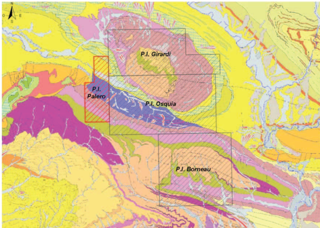
Figura 2. Geología Regional.
