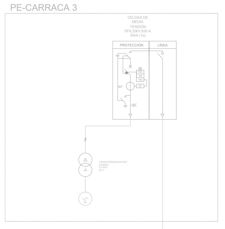
LÍNEA 5 DE PE-CARRACA 3 A CELDAS MT DE SET ELEVADORA. ALUPE 1220 KV 2427400007/Longitud= 500 m
