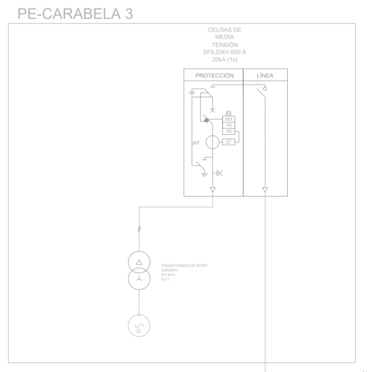
LÍNEA 4 DE PE-CARABELA 3 A CELDAS MT DE SET ELEVADORA. ALUPE 1220 KV 2427400007/Longitud= 500 m
