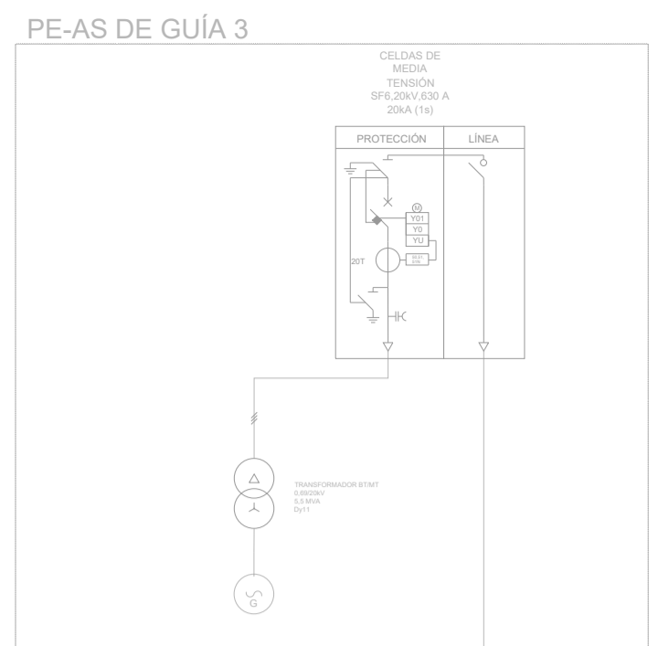
LÍNEA 1 DE PE-AS DE GUÍA 3 A CELDAS MT DE SET ELEVADORA. ALUPE 1220 KV 2427400007/Longitud= 2000 m
