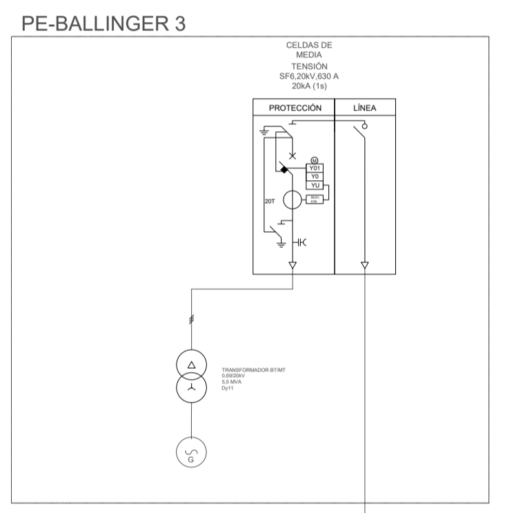
LÍNEA 3 DE PE-BALLINGER 3 A CELDAS MT DE SET ELEVADORA. ALUPE 1220 KV 2427400007/Longitud= 1000 m
