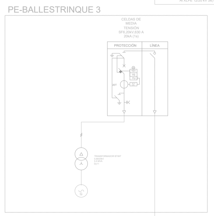
LÍNEA 2 DE PE-BALLESTRINQUE 3 A CELDAS MT DE SET ELEVADORA. ALUPE 1220 KV 2427400007/Longitud= 2000 m
