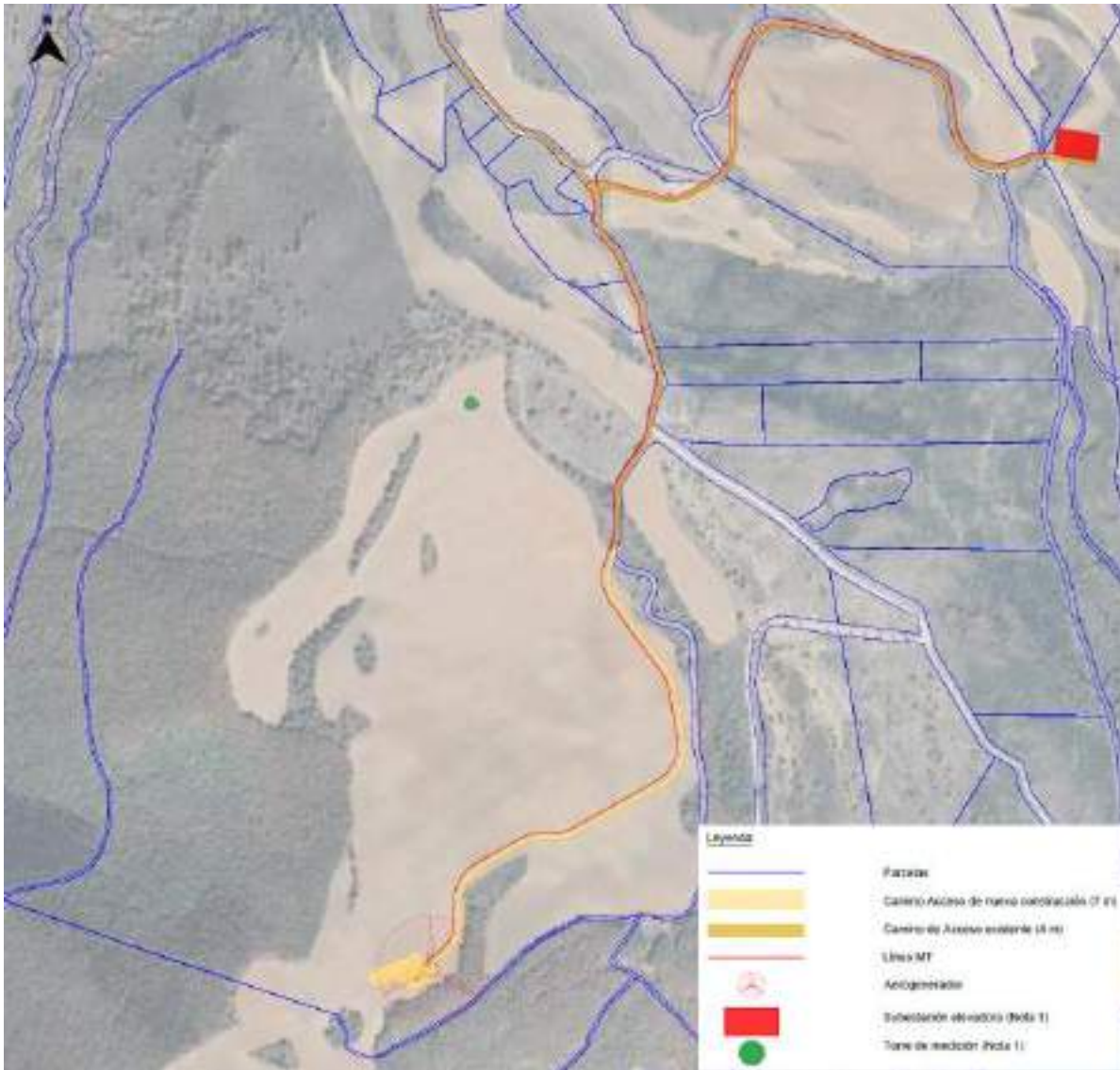
Figura 4: Layout del Parque Eólico
