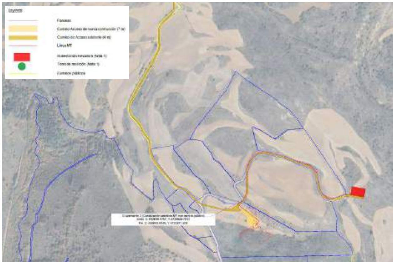
Figura 13. Afecciones del Parque Eólico a caminos públicos
