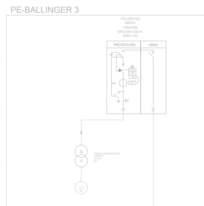
LÍNEA 3 DE PE-BALLINGER 3 A CELDAS MT DE SET ELEVADORA. AL ALPTE 12320 KV 242700000V Longitud: 1040 m
