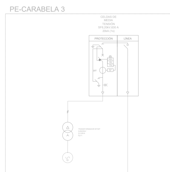
LÍNEA 4 DE PE-CARABELA 3 A CELDAS MT DE SET ELEVADORA. AL ALPTE 12320 KV 242700000V Longitud: 970 m
