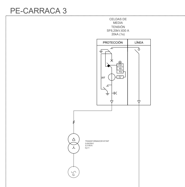
LÍNEA 5 DE PE-CARRACA 3 A CELDAS MT DE SET ELEVADORA. AL ALPTE 12320 KV 242700000V Longitud: 144 m
