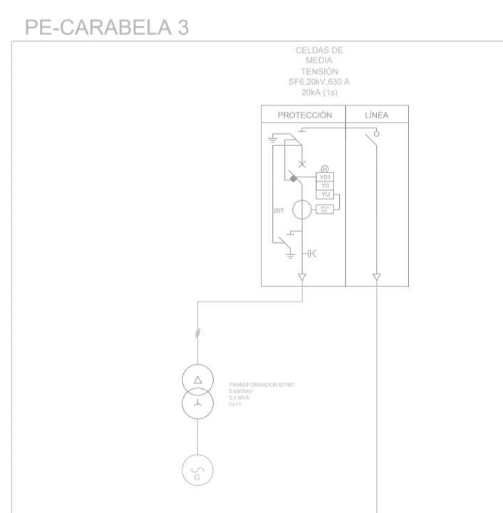
LÍNEA 4 DE PE-CARABELA 3 A CELDAS MT DE SET ELEVADORA. AL ALPE 1200 KV 240/240KV/1LUNGA/800 m
