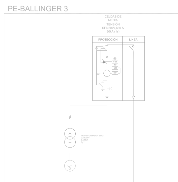
LÍNEA 3 DE PE-BALLINGER 3 A CELDAS MT DE SET ELEVADORA. AL ALPE 1200 KV 240/240KV/1LUNGA/1000 m
