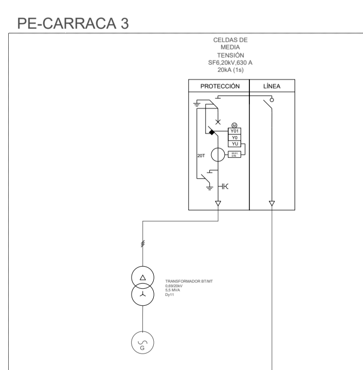
LÍNEA 5 DE PE-CARRACA 3 A CELDAS MT DE SET ELEVADORA. AL ALPE 1200 KV 240/240KV/1LUNGA/500 m
