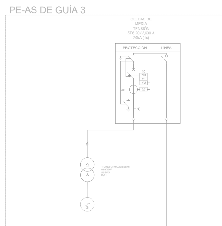
LÍNEA 1 DE PE-AS DE GUÍA 3 A CELDAS MT DE SET ELEVADORA. AL ALPE 1200 KV 240/240KV/1LUNGA/2000 m
