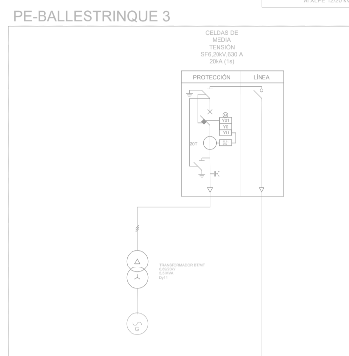
LÍNEA 2 DE PE-BALLESTRINQUE 3 A CELDAS MT DE SET ELEVADORA. AL ALPE 1200 KV 240/240KV/1LUNGA/1200 m
