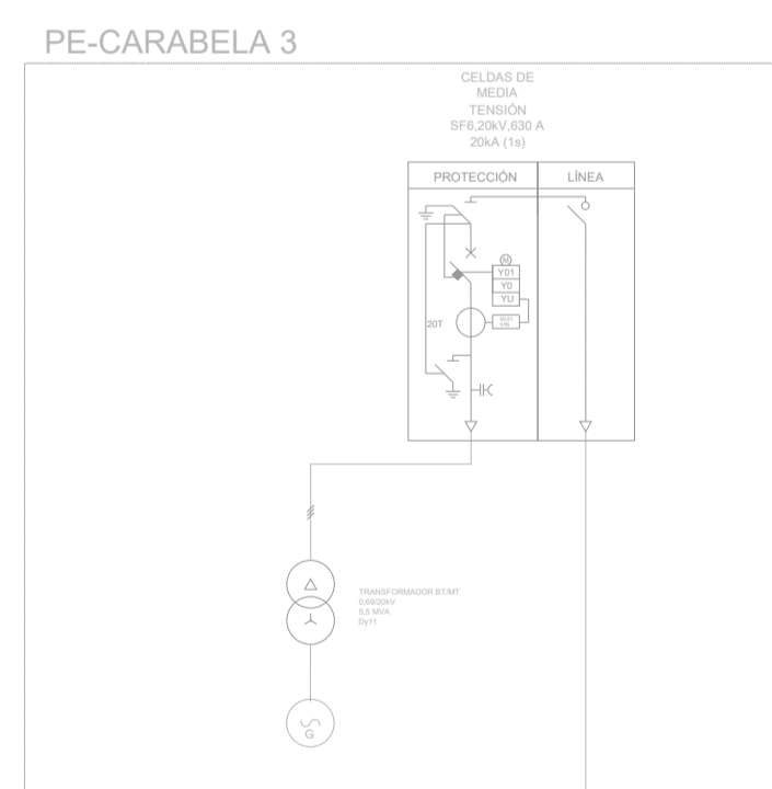
LÍNEA 4 - DE PE-CARABELA 3 A CELDAS MT DE SET ELEVADORA. - ALUPE 1200 KV 2x2 Conductores/Línea=500 m
