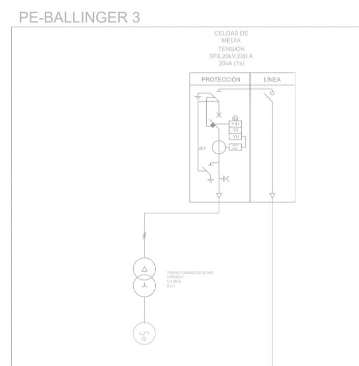
LÍNEA 3 - DE PE-BALLINGER 3 A CELDAS MT DE SET ELEVADORA. - ALUPE 1200 KV 2x2 Conductores/Línea=1000 m
