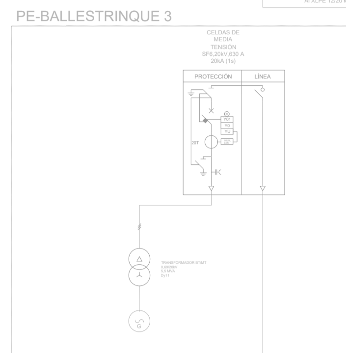
LÍNEA 2 - DE PE-BALLESTRINQUE 3 A CELDAS MT DE SET ELEVADORA. - ALUPE 1200 KV 2x2 Conductores/Línea=2000 m
