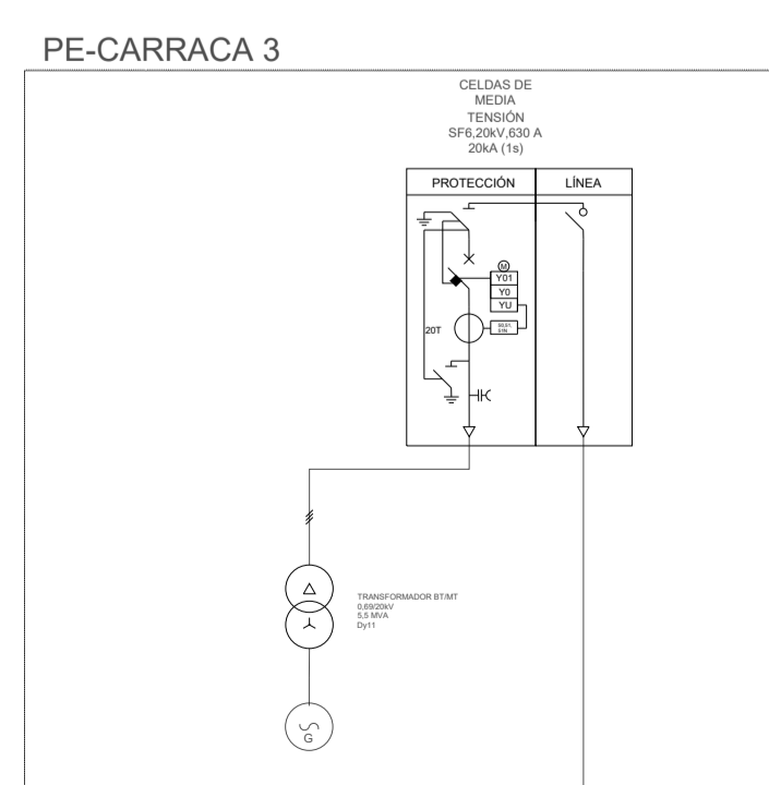
LÍNEA 5 - DE PE-CARRACA 3 A CELDAS MT DE SET ELEVADORA. - ALUPE 1200 KV 2x2 Conductores/Línea=500 m
