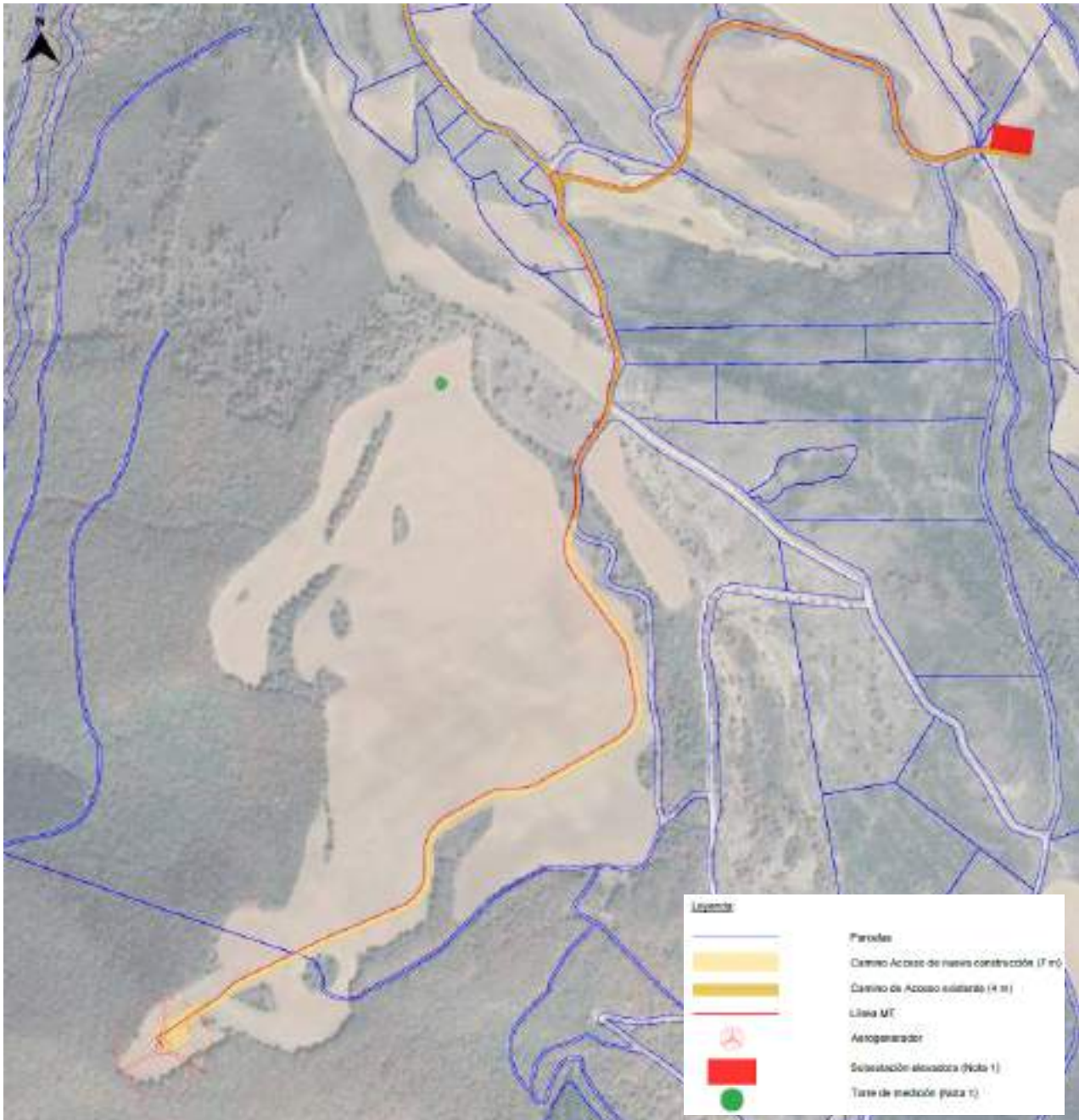
Figura 4: Layout del Parque Eólico
