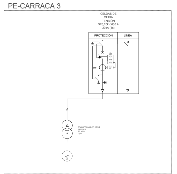
LÍNEA 5 DE PE-CARRACA 3 A CÉLULAS MT DE SET ELEVADORA. AL ALPTE 1220 KV 2427000000/longitud= 500 m
