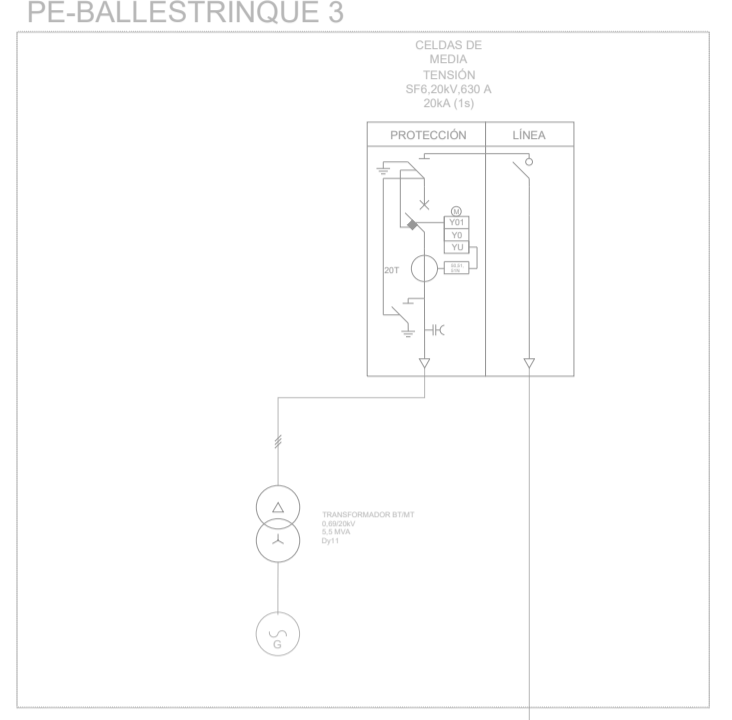
LÍNEA 2 DE PE-BALLESTRINQUE 3 A CÉLULAS MT DE SET ELEVADORA. AL ALPTE 1220 KV 2427000000/longitud= 2000 m
