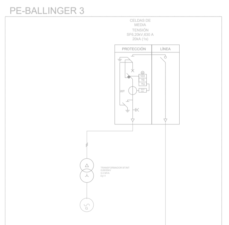
LÍNEA 3 DE PE-BALLINGER 3 A CÉLULAS MT DE SET ELEVADORA. AL ALPTE 1220 KV 2427000000/longitud= 1000 m
