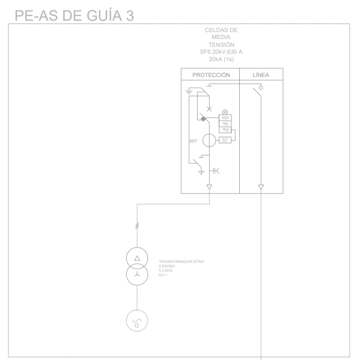
LÍNEA 1 DE PE-AS DE GUÍA 3 A CÉLULAS MT DE SET ELEVADORA. AL ALPTE 1220 KV 2427000000/longitud= 2000 m
