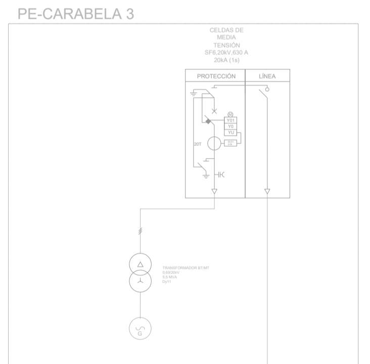
LÍNEA 4 DE PE-CARABELA 3 A CÉLULAS MT DE SET ELEVADORA. AL ALPTE 1220 KV 2427000000/longitud= 500 m
