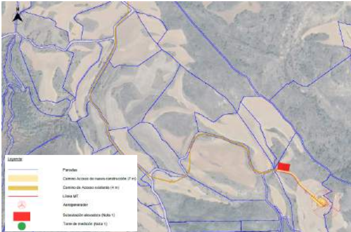
Figura 4: Layout del Parque Eólico
