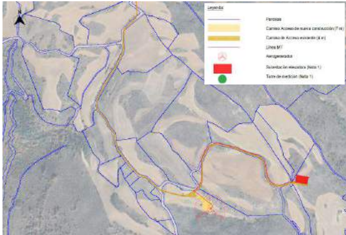
Figura 4: Layout del Parque Eólico
