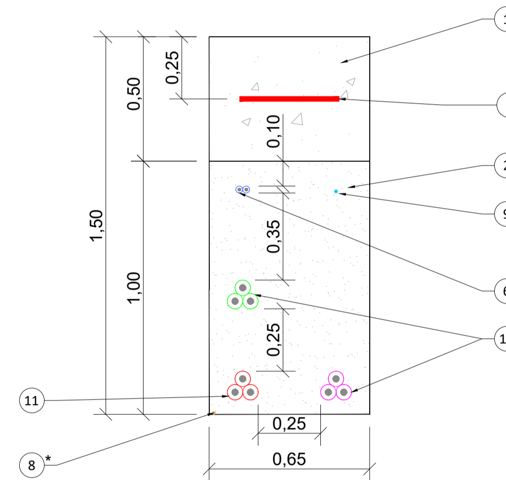
3 LÍNEAS, CABLE MT 1 LÍNEA, CABLE BT CABLE COMUNICACIÓN ENTERRADO DIRECTO
