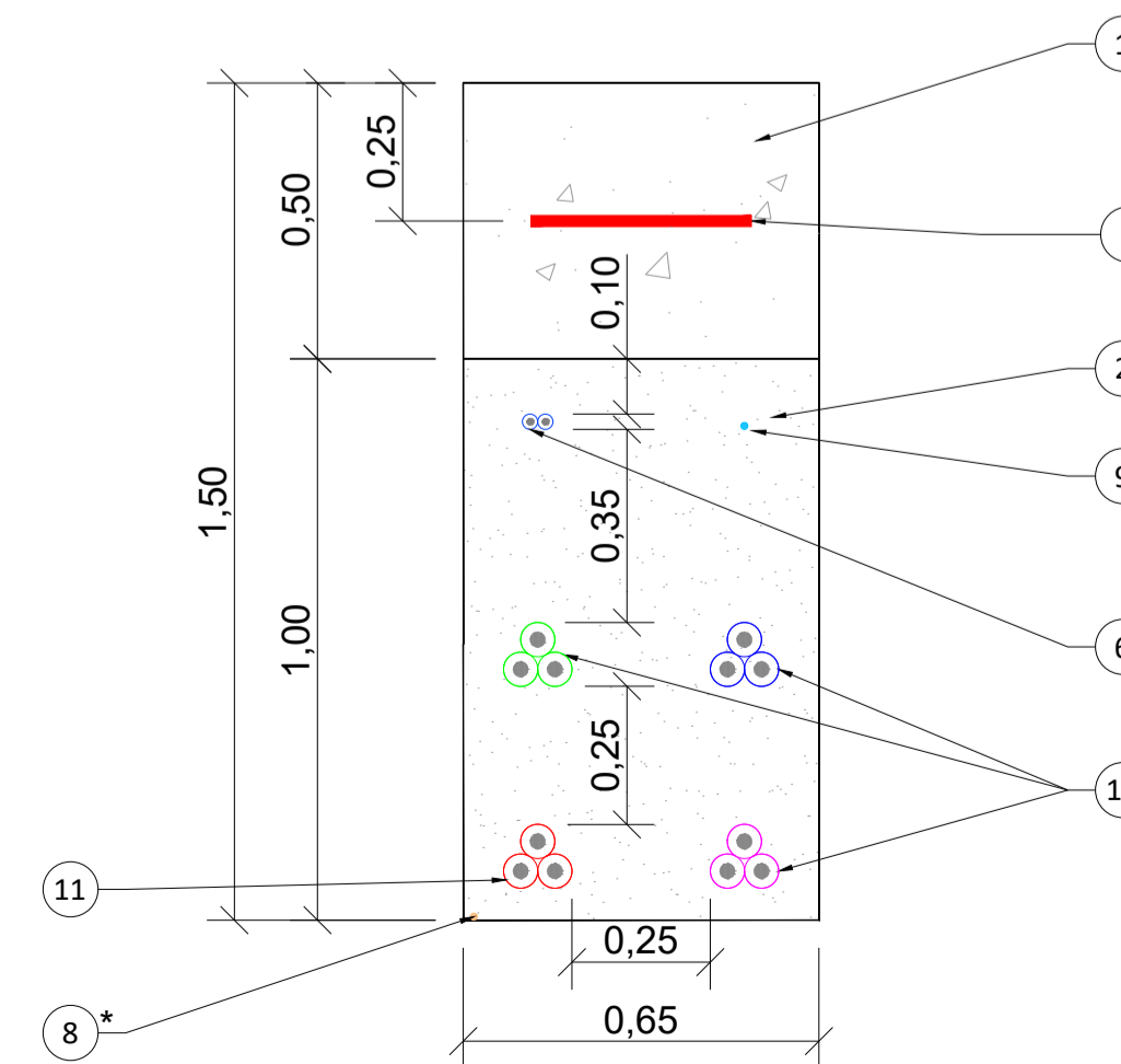
4 LÍNEAS, CABLE MT 1 LÍNEA, CABLE BT CABLE COMUNICACIÓN ENTERRADO DIRECTO
