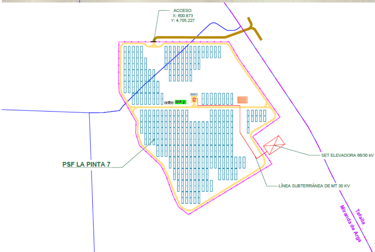
Figura 19: Instalación FV.
