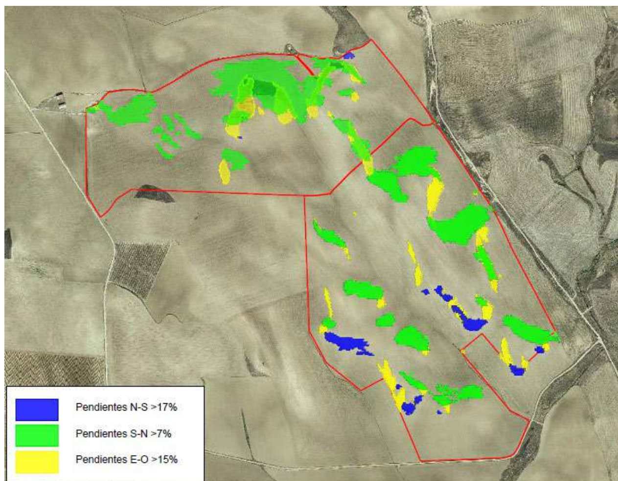
Figura 4: Pendientes.
