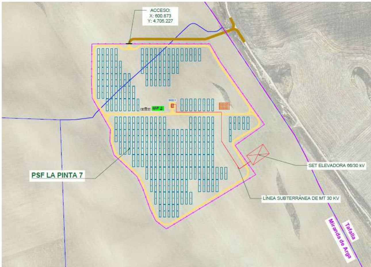
Figura 14: Caminos existentes.
