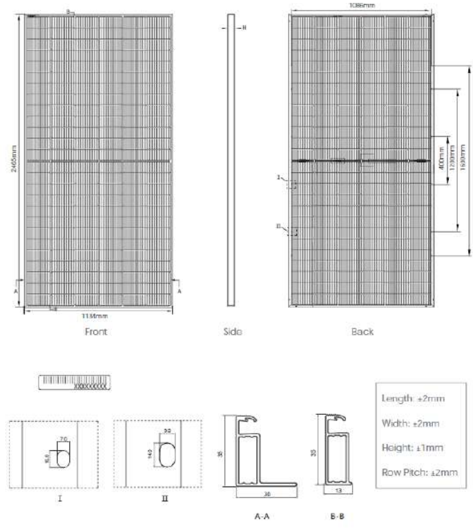
Figura 20: Dimensiones del Módulo.
