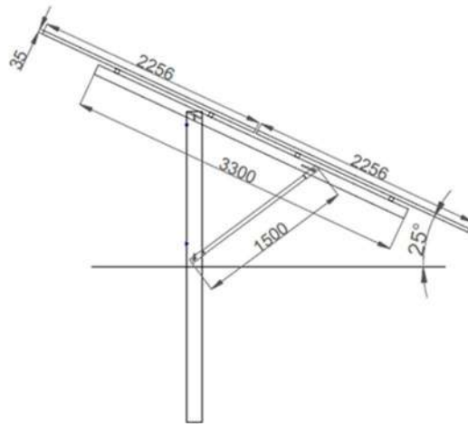
Figura 8.- Estructura soporte.
