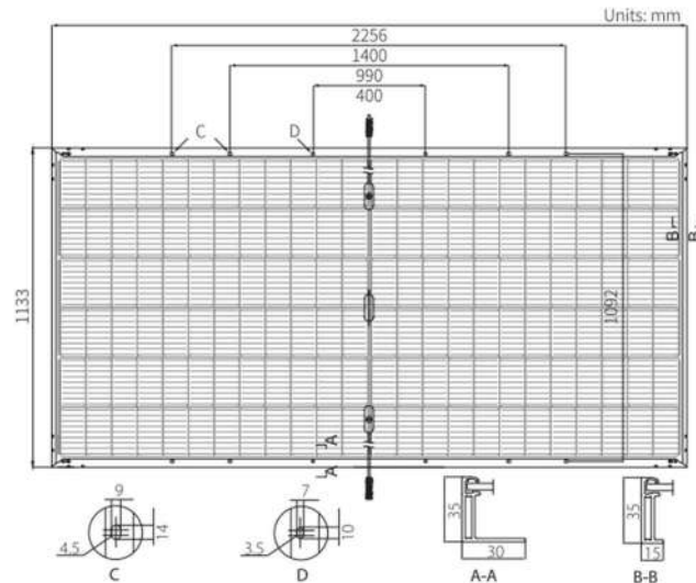
Figura 7.- Módulo fotovoltaico.
