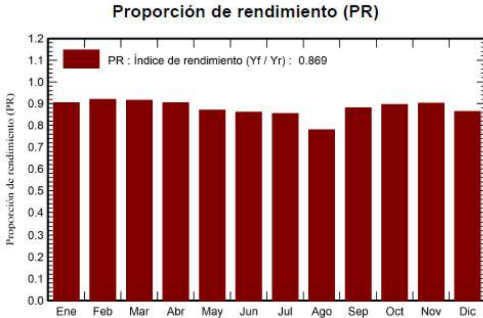
Ilustración 7 : Performance ratio.
