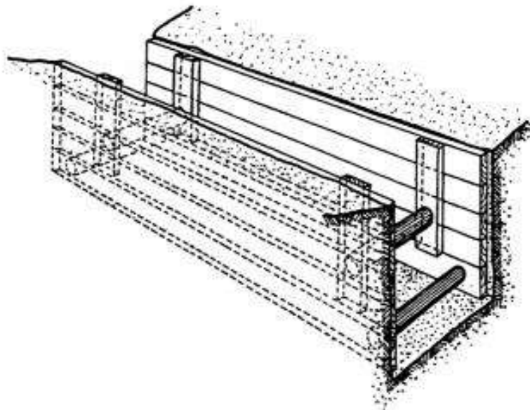
ENTIBACIÓN CUAJADA
