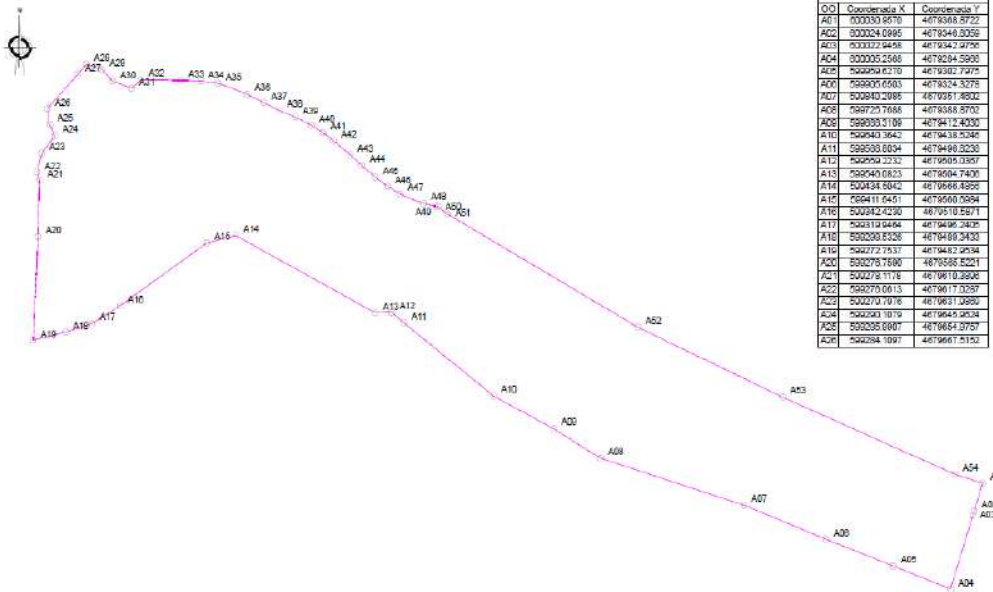
Ilustración 3 : Superficie instalación.
