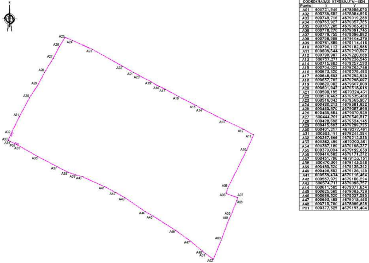
Ilustración 3 : Superficie instalación.
