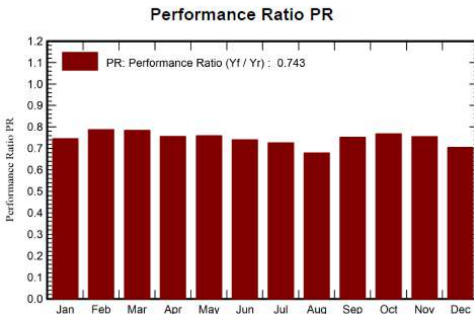
Ilustración 7 : Performance ratio.
