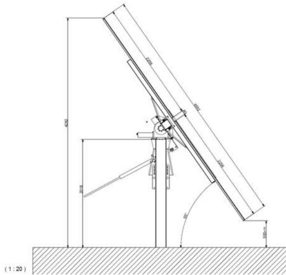
Ilustración 5: Estructura soporte
