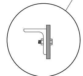
DETALLE FIJACIÓN ENTRE ÁNGULO Y PIQUETA
