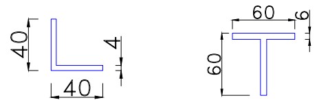
Escala 1:5 Cotas en mm
