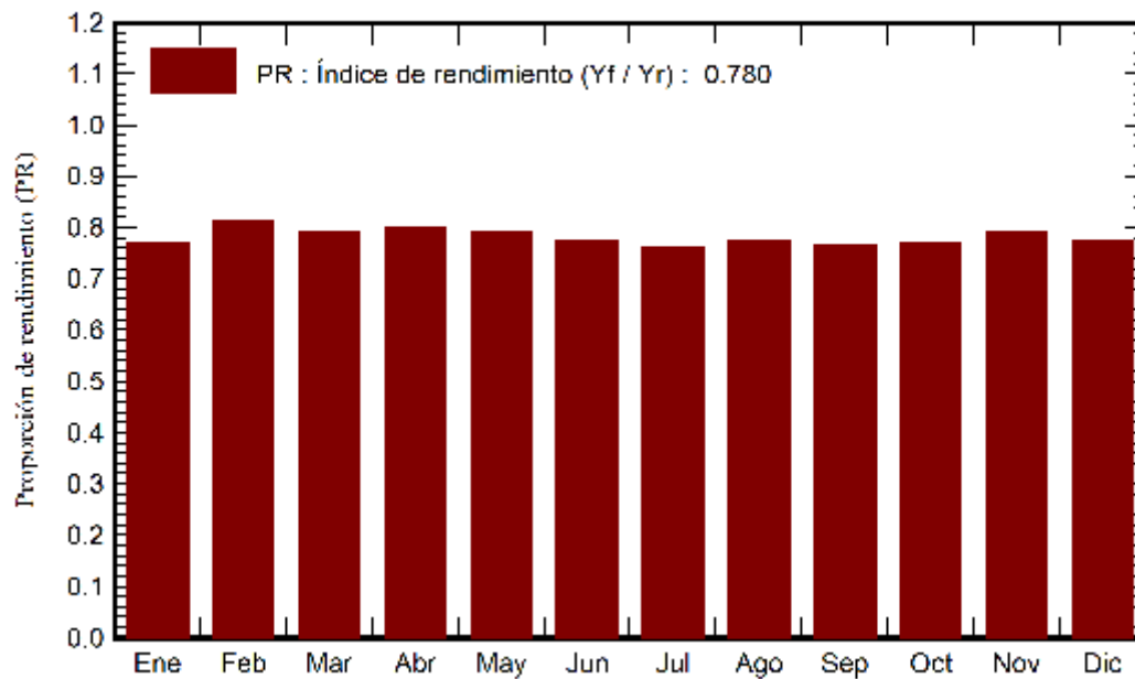
Ilustración 7 : Performance ratio.
