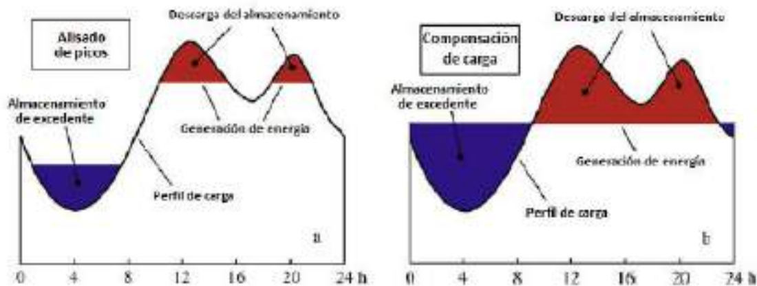
Figura 7. Aplicación de sistemas de almacenamiento en sistemas fotovoltaicos.
