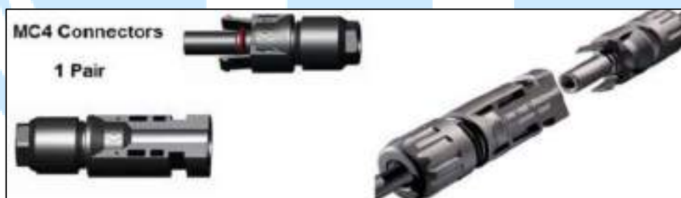
Figura 20. Conector MC4 del cable solar.
