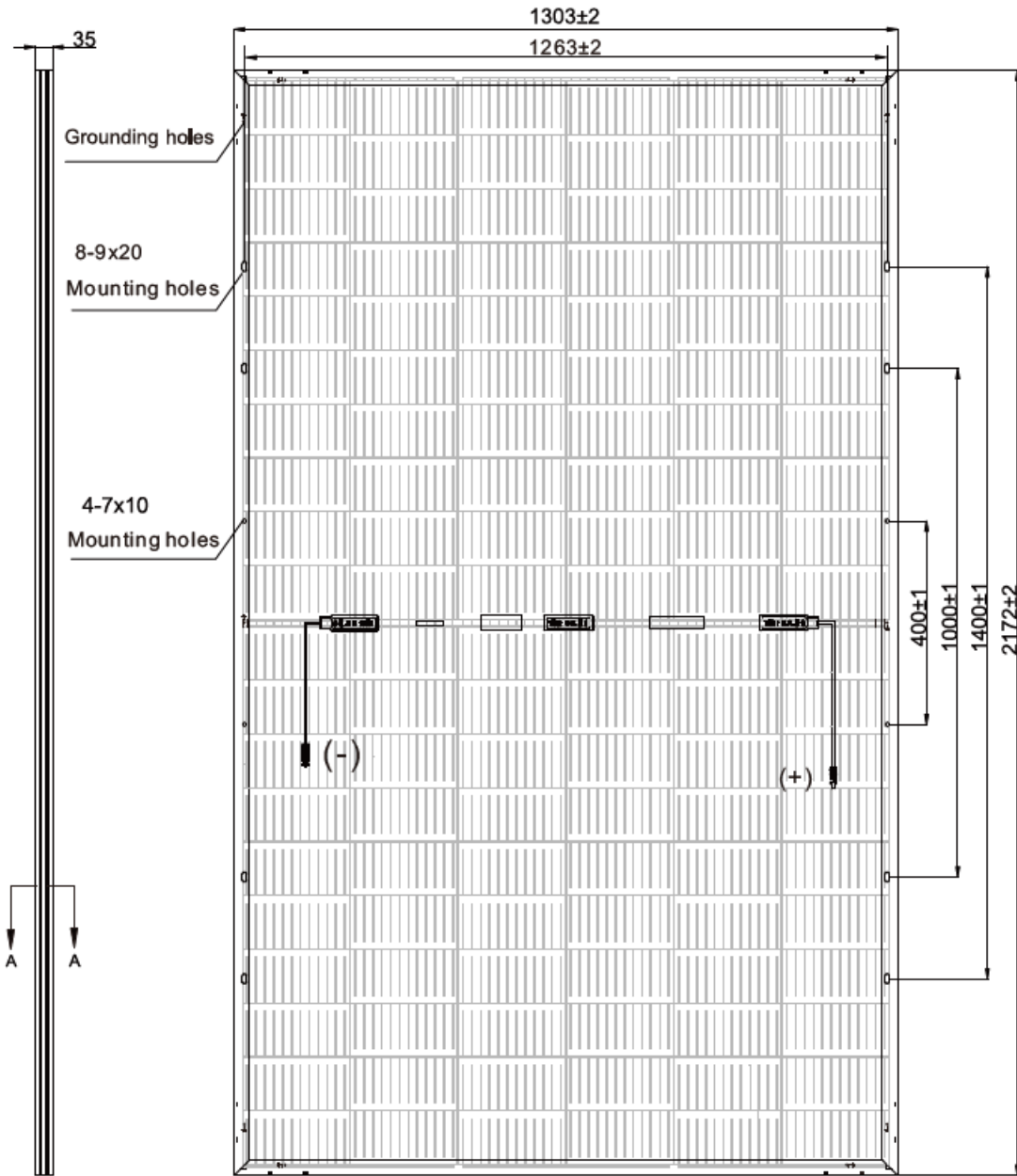
Figura 15. Dimensiones del módulo fotovoltaico.
