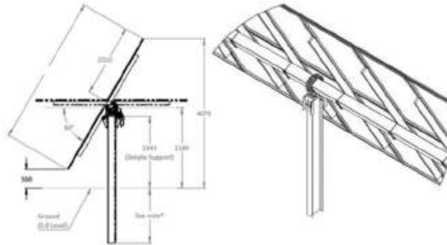
Figura 18. Perfil seguidor solar y detalle del eje.
