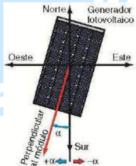
Figura 6. Representación de la orientación o azimut de un panel fotovoltaico
