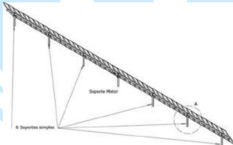
Figura 17. Perfiles de cimentación estructura seguidor.
