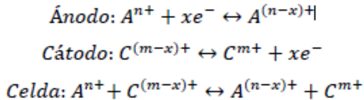
Figura 9. Reacción química entre ánodo y cátodo del sistema de almacenamiento de energía.
