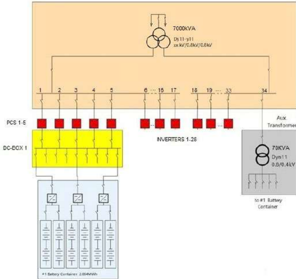
Figura 12. Configuración de sistema de almacenaje OPCIONAL
