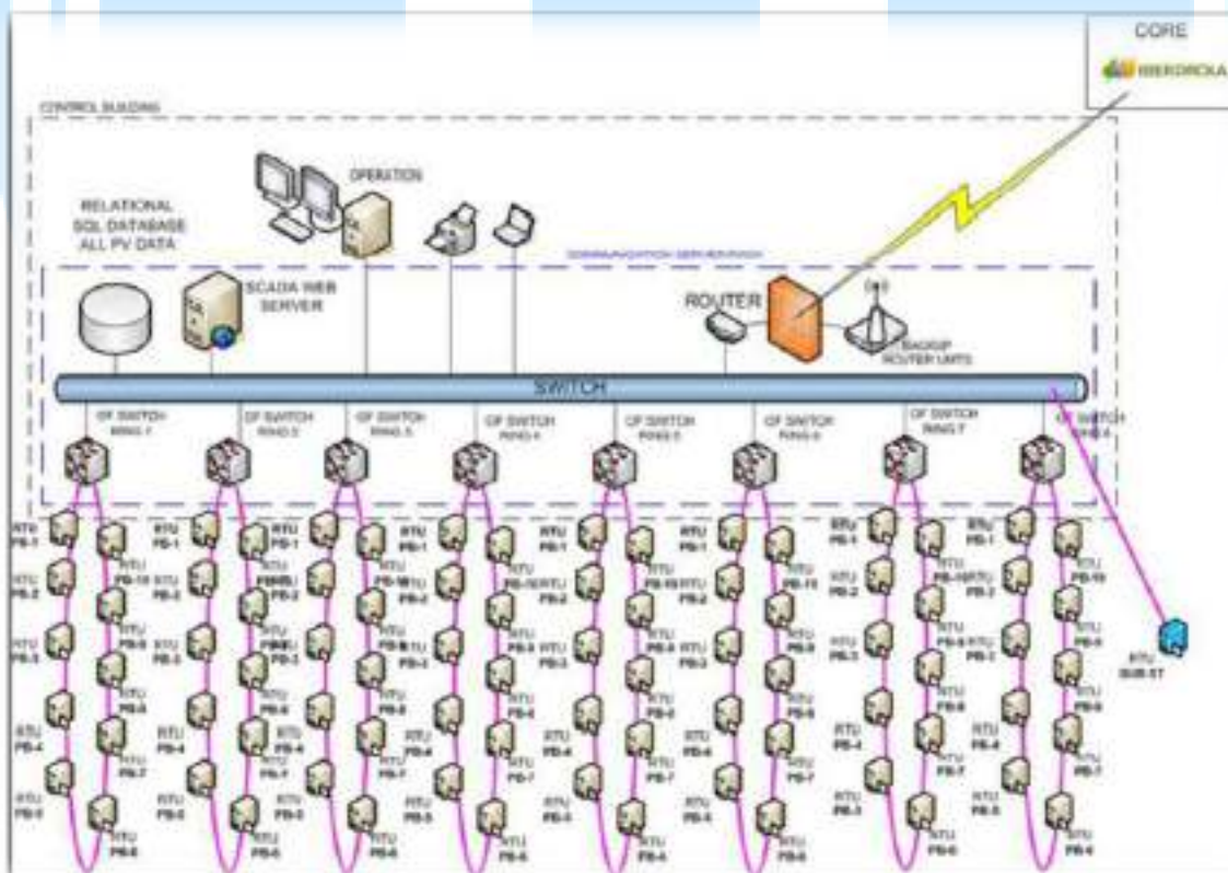
Figura 26. Conexión de equipo SCADA.
