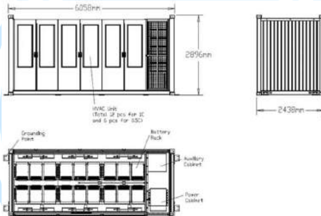
Figura 11. Dimensiones típicas de un sistema BESS.
