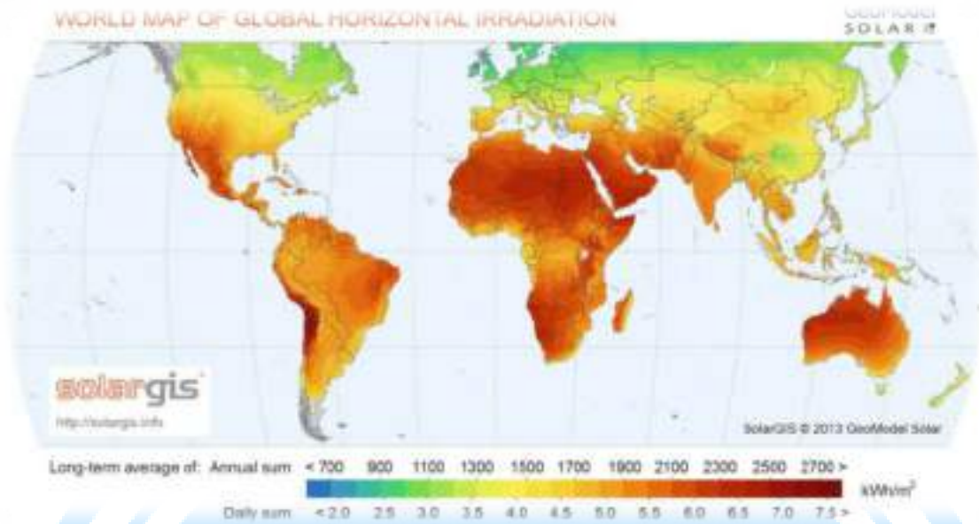
Figura 3. Irradiación media diaria y anual en el mundo. Vía SolarGIS.
