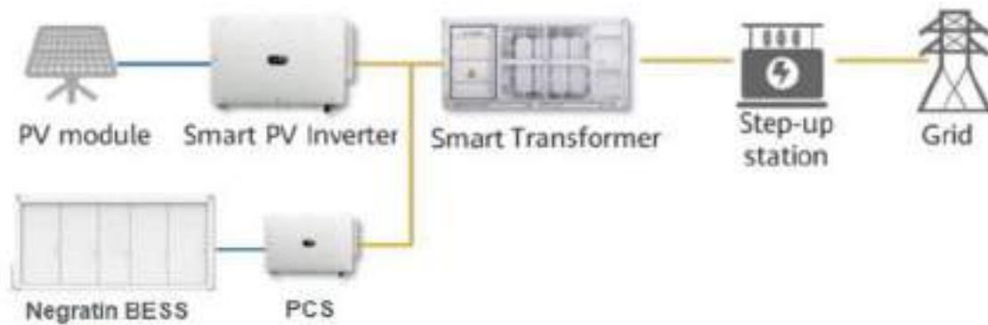
Figura 10. Implementación del sistema BESS en la línea de producción de energía fotovoltaica.
