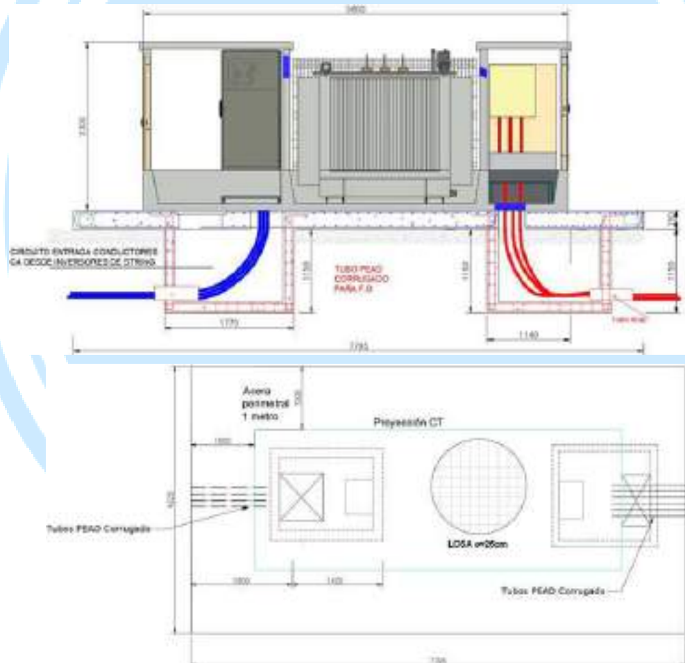
Figura 24. Ejemplo de cimentación CT
