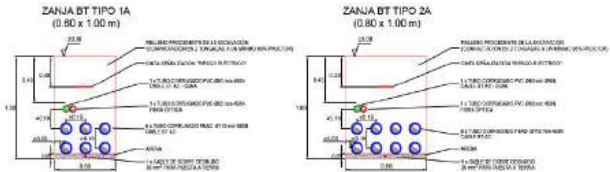
Figura 21. Representación tipos de zanjas BT.
