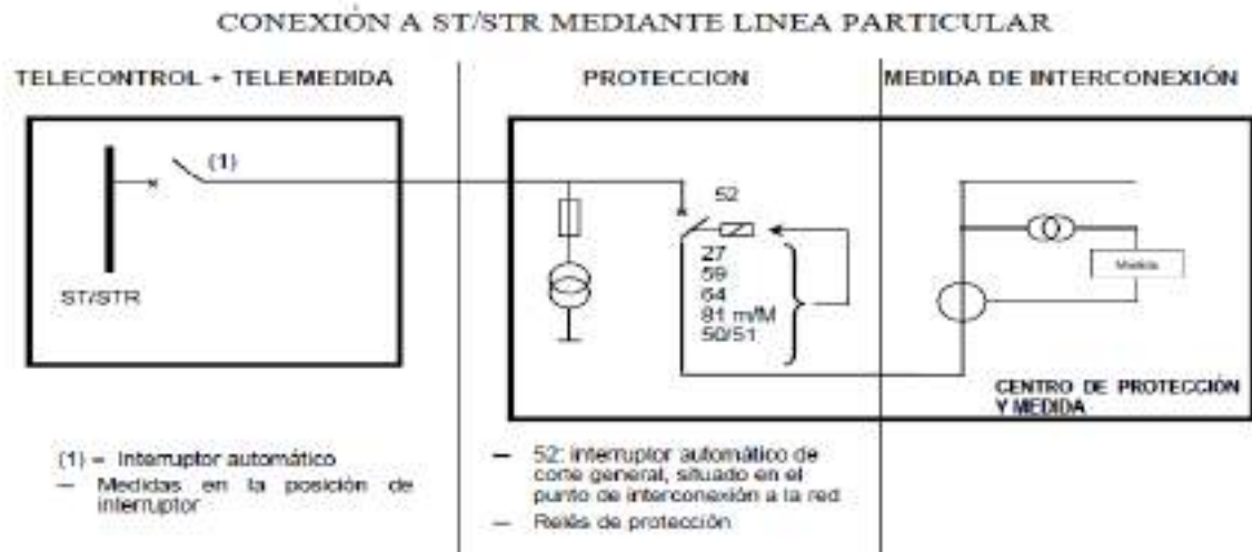
Figura 23. Diagrama unifilar de la conexión a la subestación
