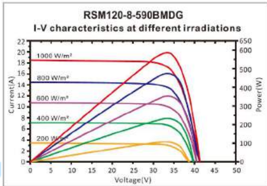
Figura 13. Gráfica I-V para diferente irradiación incidente sobre el módulo fotovoltaico.
