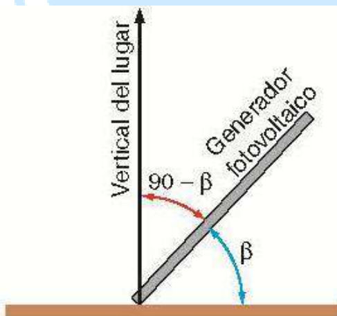
Figura 5. Representación de la inclinación de un panel fotovoltaico.
