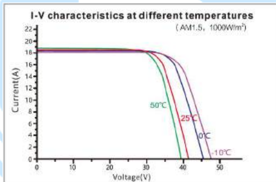
Figura 14. Gráfica I-V para diferentes temperaturas en el módulo fotovoltaico.
