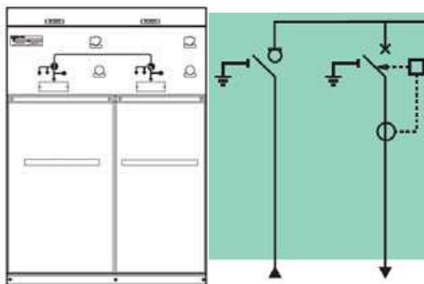
Alzado y esquema de celdas.
