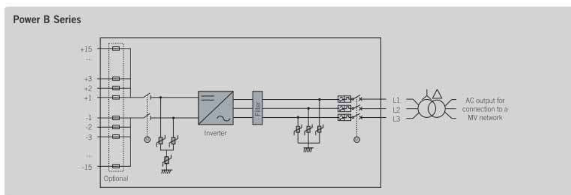
Esquema unifilar genérico
