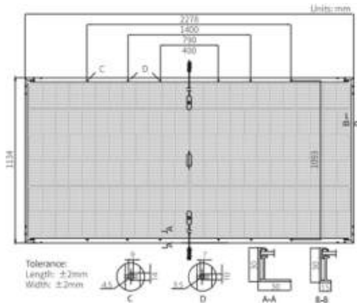
Figura 9.- Módulo fotovoltaico.
