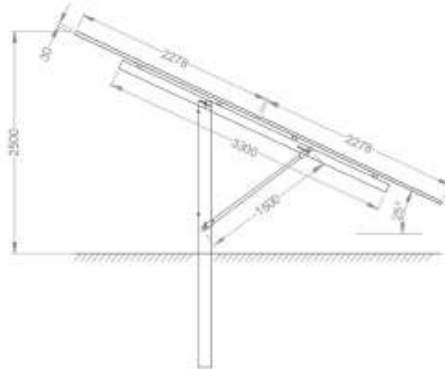
Figura 10.- Estructura soporte.
