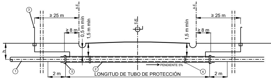
SECCIÓN TIPO. AUTOPISTAS, AUTOVÍAS Y VÍAS RÁPIDAS
