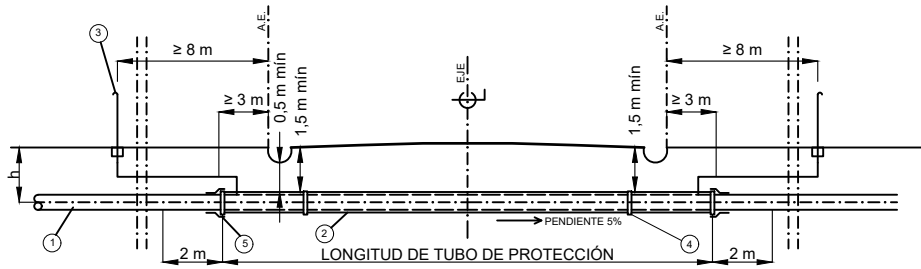
SECCIÓN TIPO. CARRETERAS
