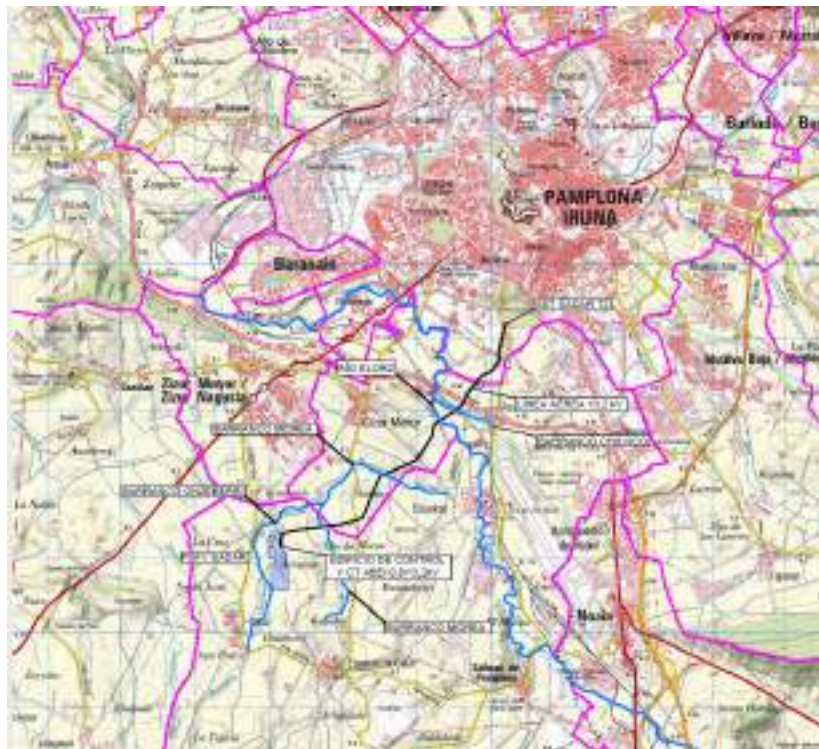
Imagen 1. Ubicación de la planta PSFV Sadar y su línea de evacuación.
