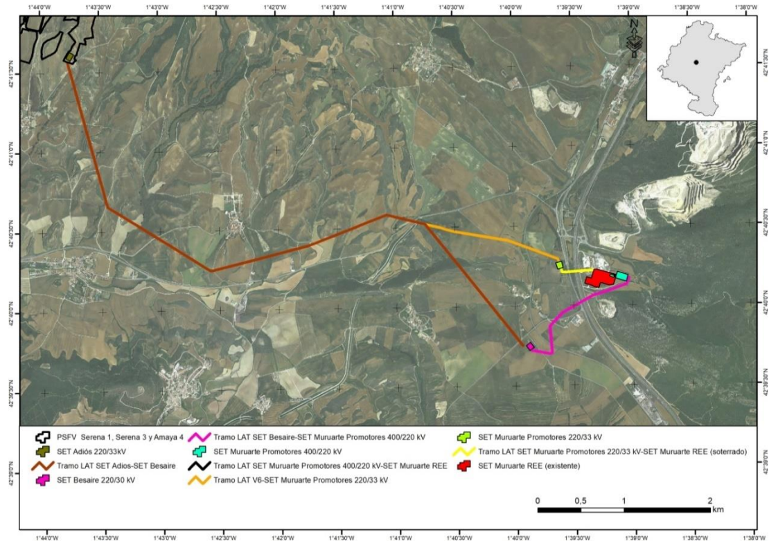
Foto 15. Fotografía aérea de ubicación de SET y LAT de evacuación.
