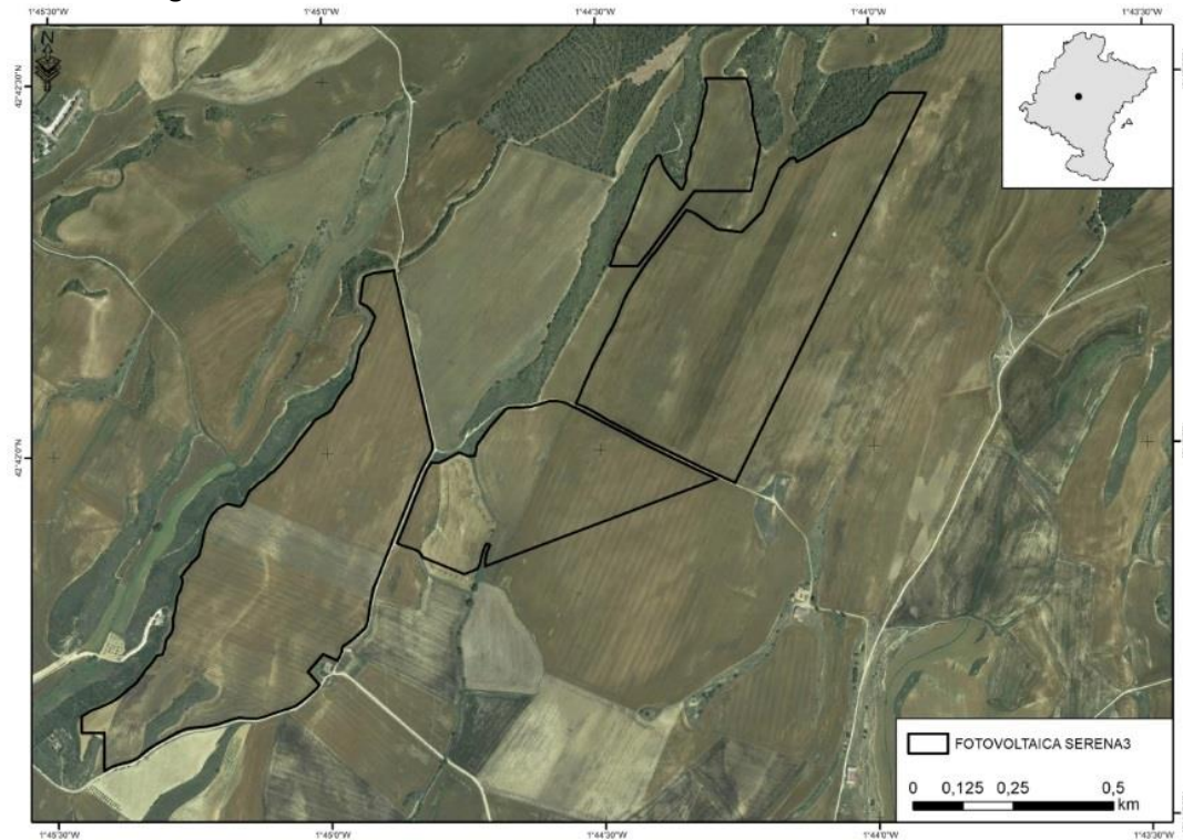
Foto 7. Fotografía aérea de Serena 3.
