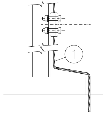
CONEXIÓN MALLA DE TIERRA A ESTRUCTURA
