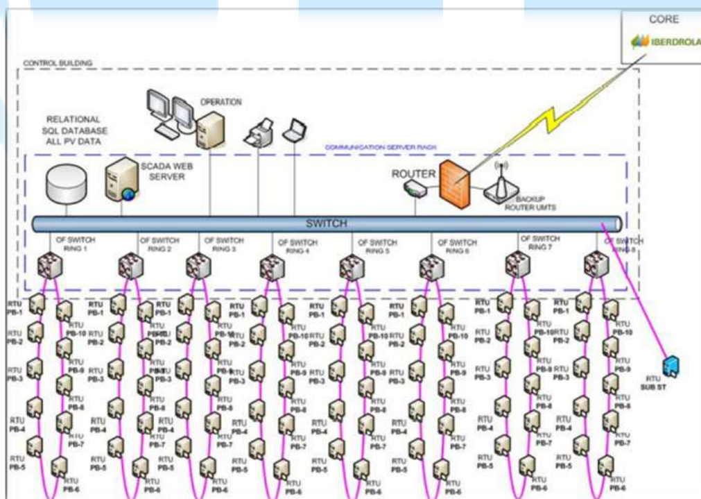
Figura 27. Conexión equipo SCADA.
