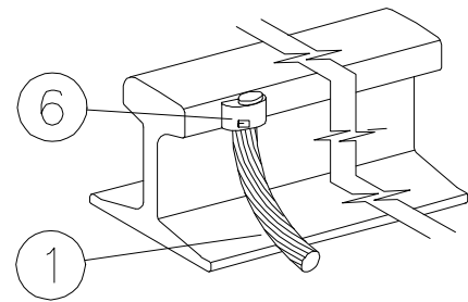
SOLDADURA ALUMINOTÉRMICA A CARRIL
