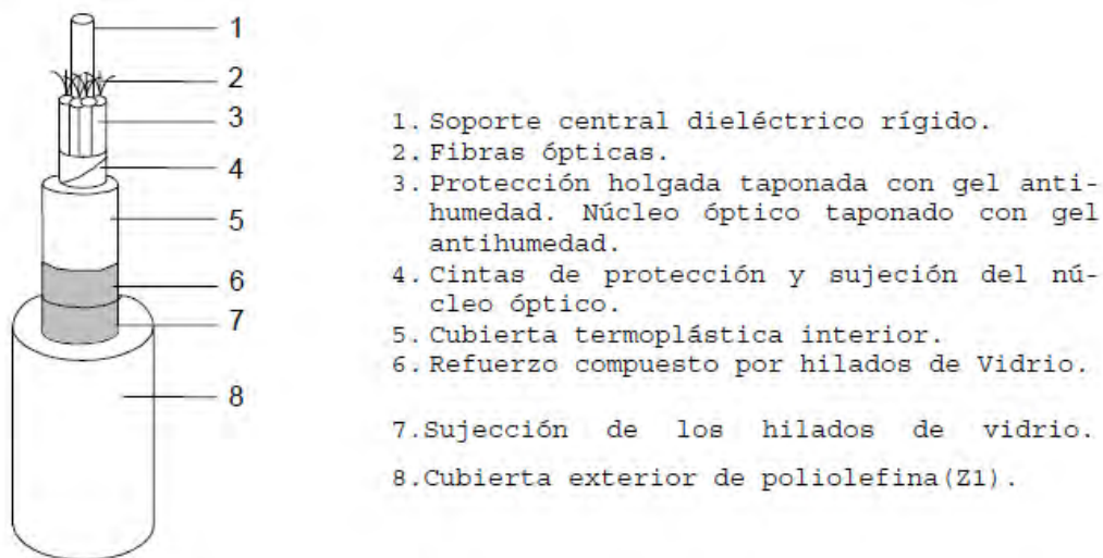
Fig.- Constitución típica del cable óptico subterráneo tipo OSGZ1
