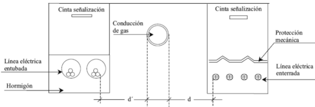
Figura 22: Detalles de paralelismo y conducciones (ITC-LAT 06).
