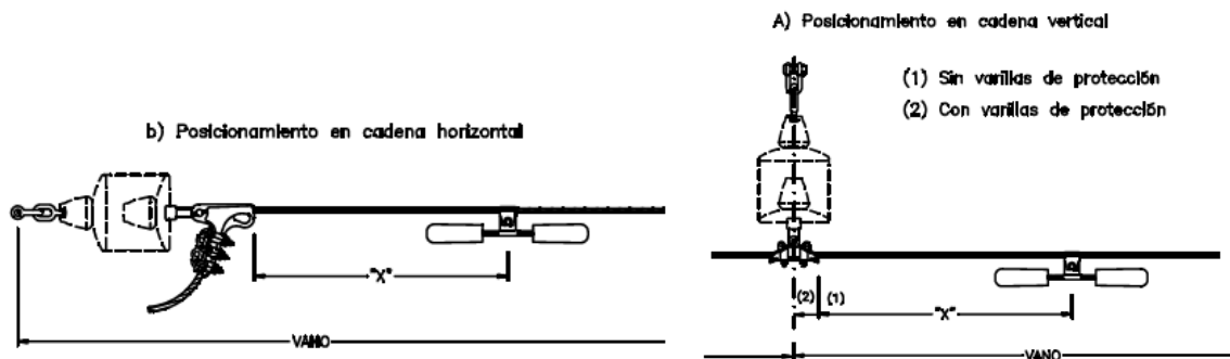
Figura 15: Posicionamiento Antivibrador.
