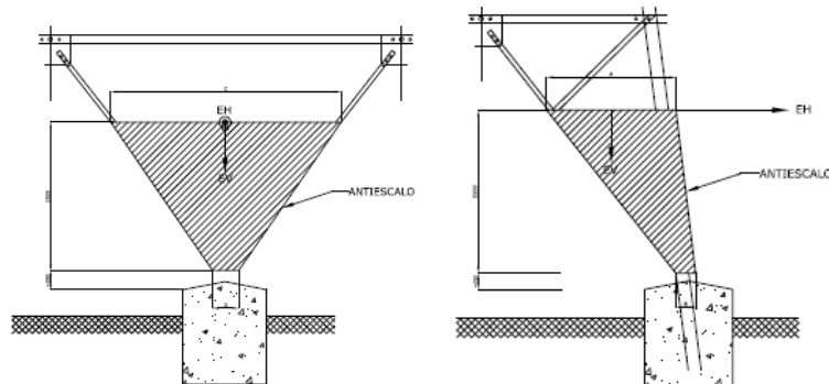
Figura 16: Sistema Antiescalo apoyos Tetrabloque.
