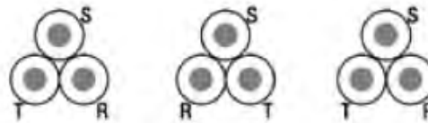
Figura 17: Colocación de cables en tresbolillo.
