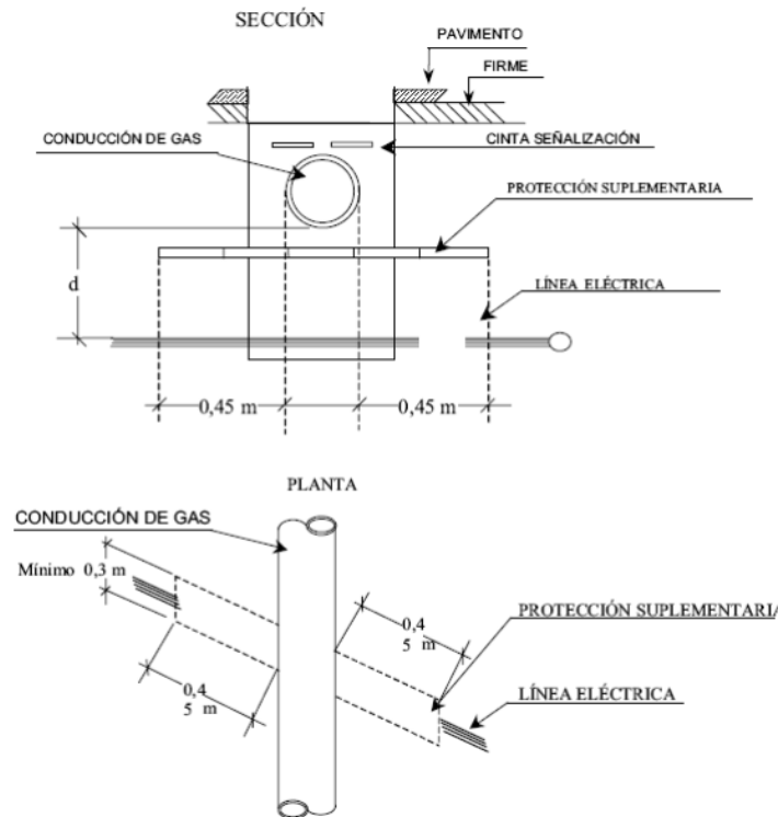
Figura 20: Detalles de cruzamiento y conducciones (ITC-LAT 06).
