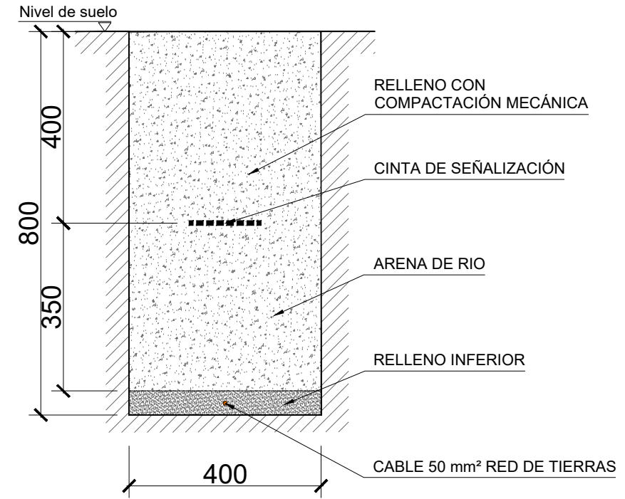
ZANJA TIERRA CENTRO DE TRANSFORMACIÓN
