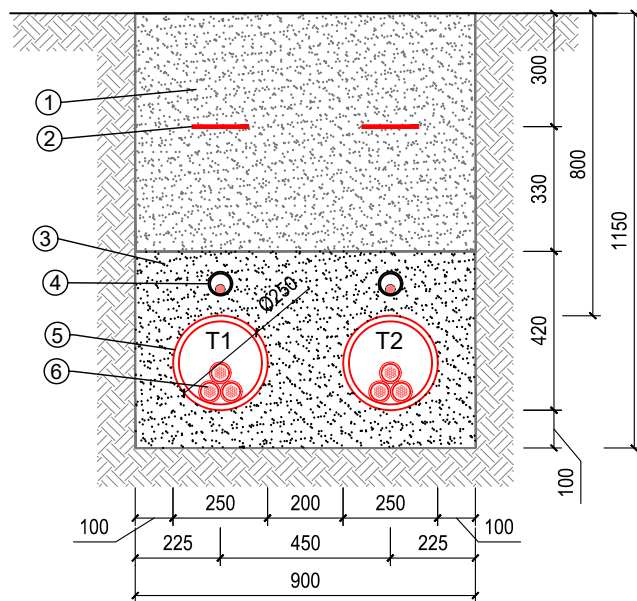
SECCIÓN TIPO ZANJA ENTUBADA 2 Circuitos
