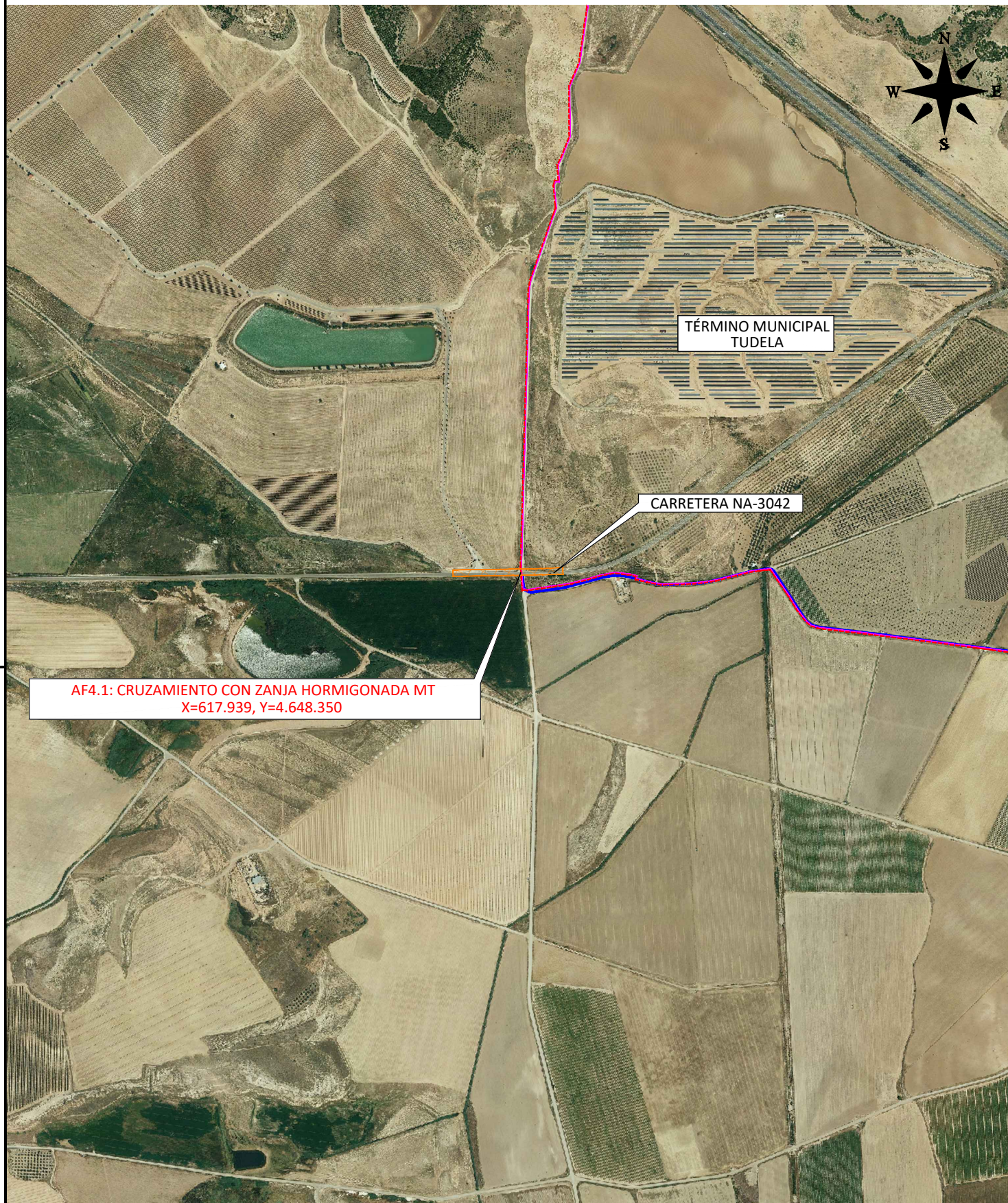
PLANTA DETALLE (Escala 1/10.000)
