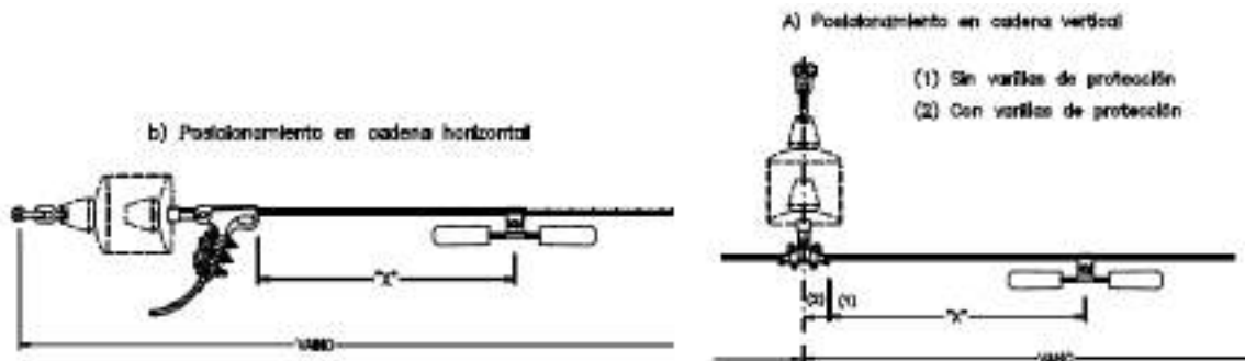
Figura 14: Posicionamiento Antivibrador.
