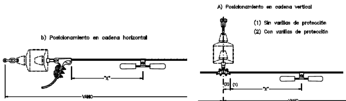
Figura 14: Posicionamiento Amortiguador.
