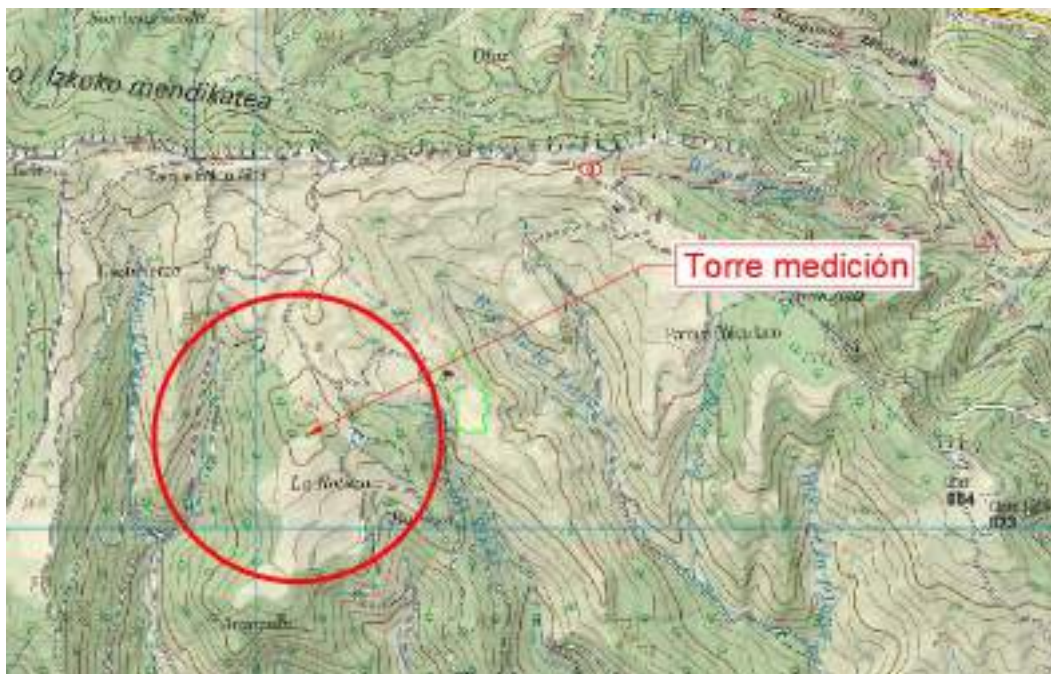
Figura 24: Localización torre de medición.
