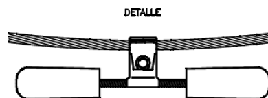
Figura 13: Amortiguador Stockbridge.
