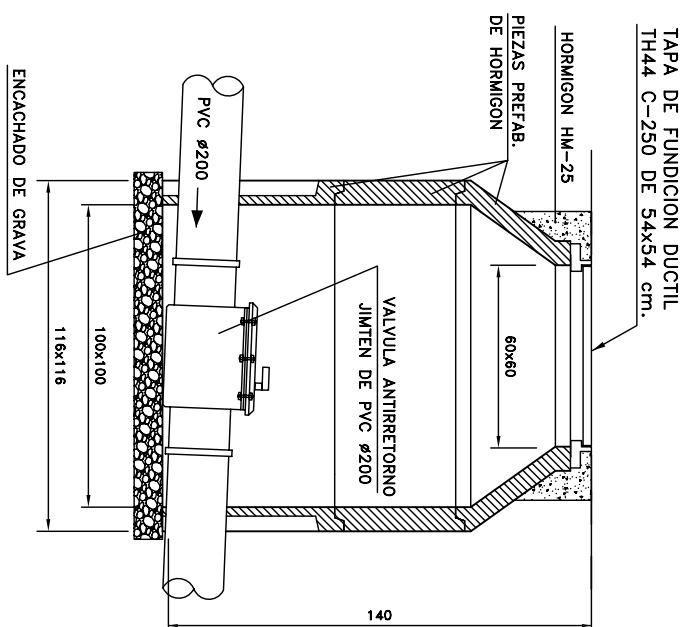
ARQUETA TIPO 2
