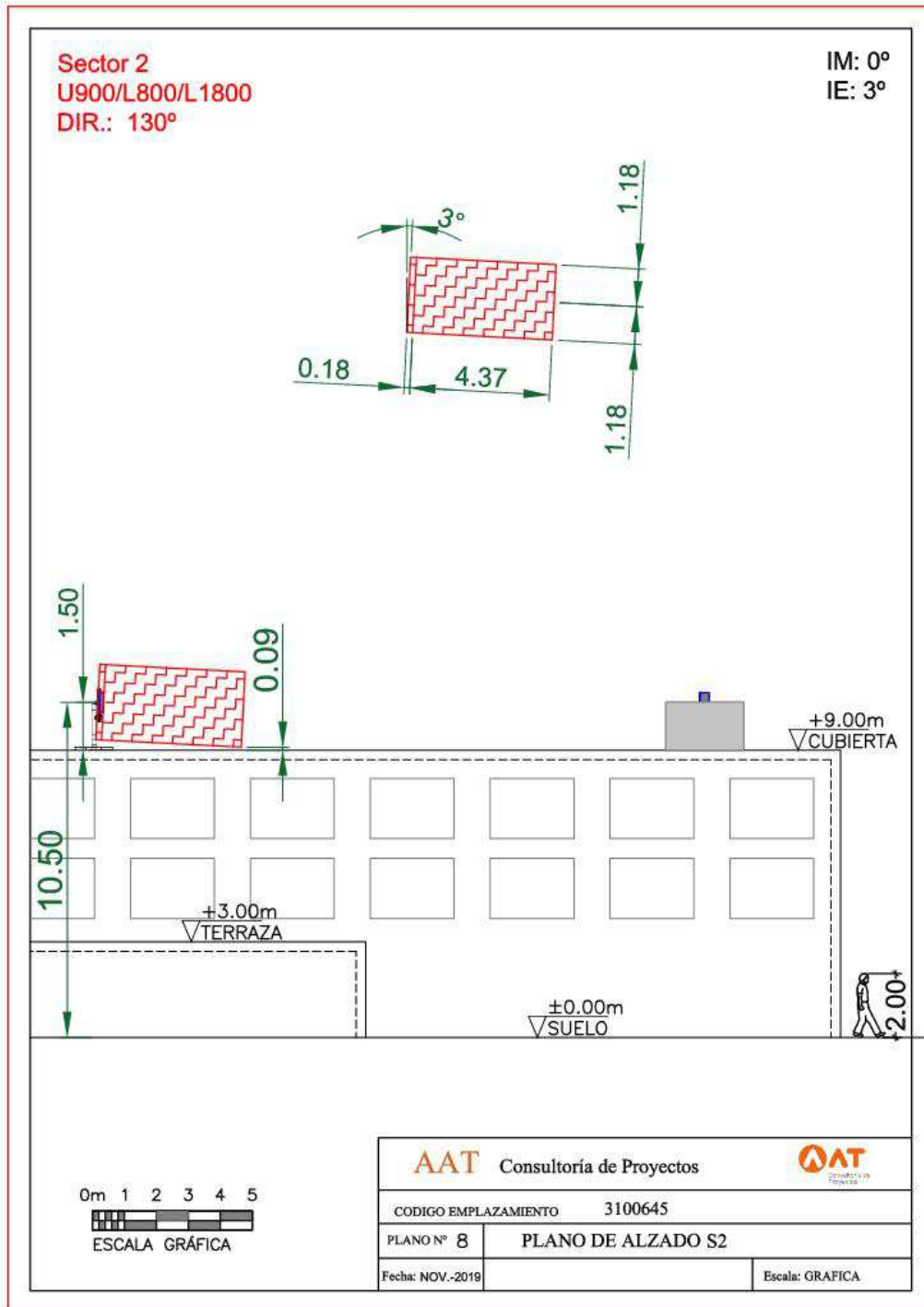
Alzado general de la instalación
