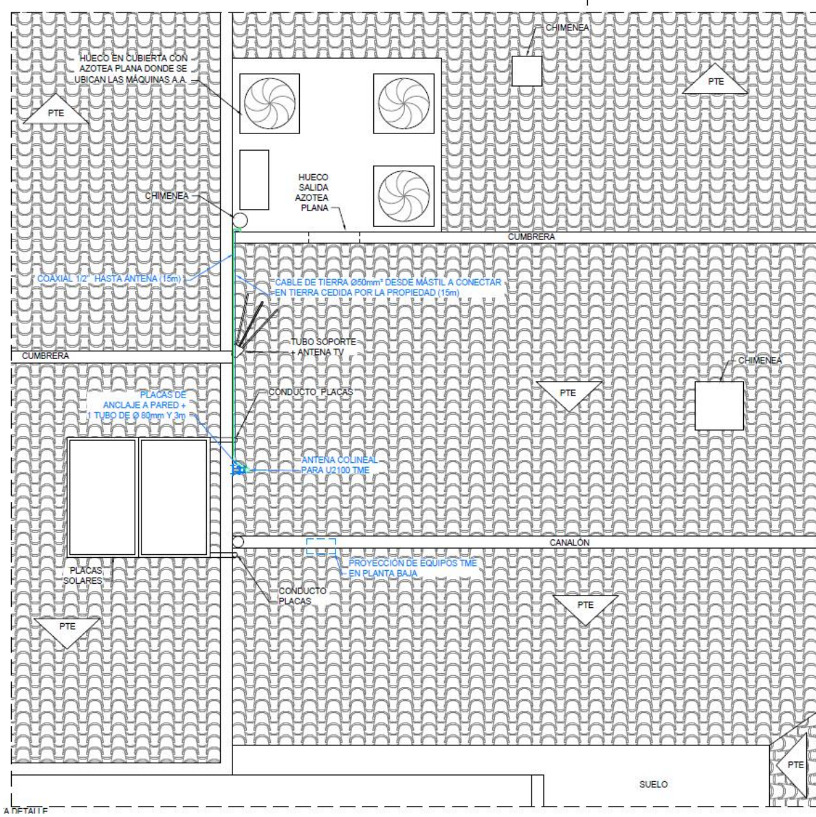
Planta de cubierta de la instalación
