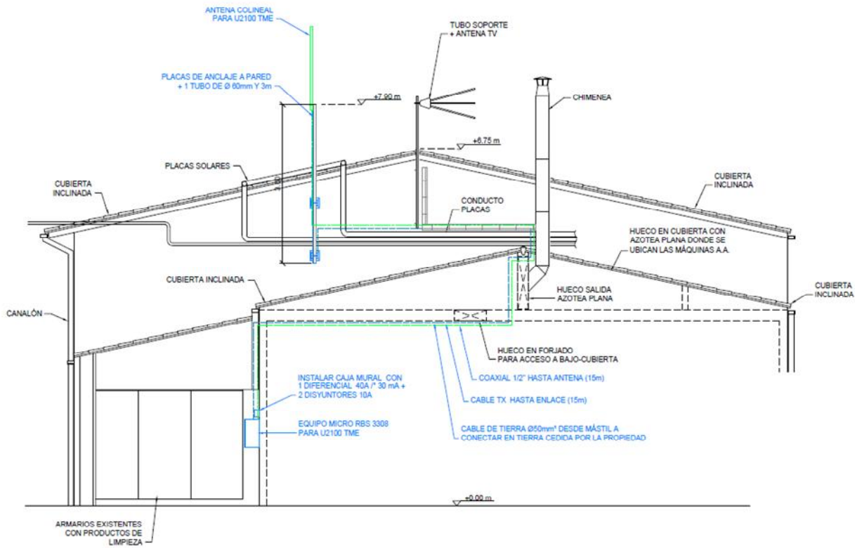
Alzado general de la instalación
