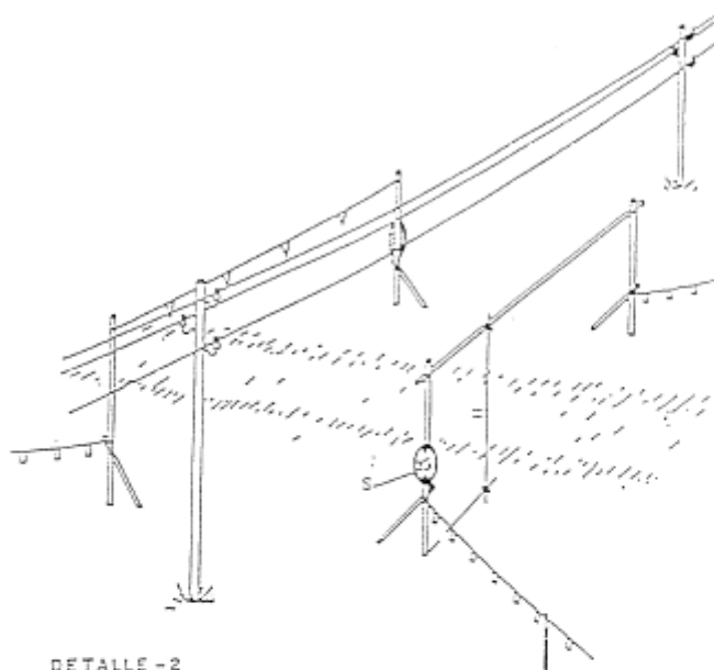
DETALLE - 2
