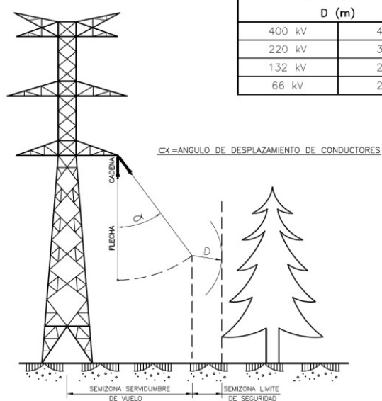
Distancia a arbolado
