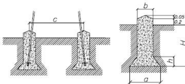
Cimentación tetrabloque (cuadrada con cueva)
