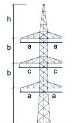
Tipos de apoyos
