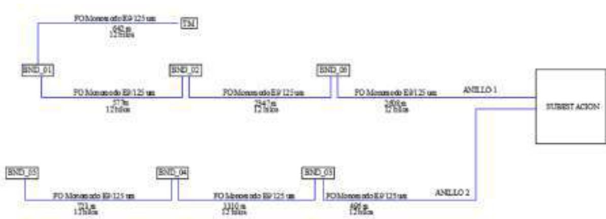
Imagen 14 Esquema de comunicaciones
