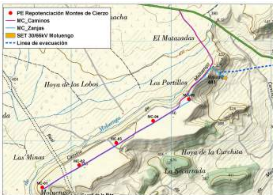
Imagen 2. Implantación de infraestructuras permanentes del parque eólico
