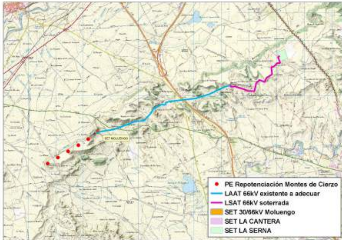
Imagen 3. Parque Eólico Repotenciación Montes de Cierzo y sistema de evacuación sobre topográfico
