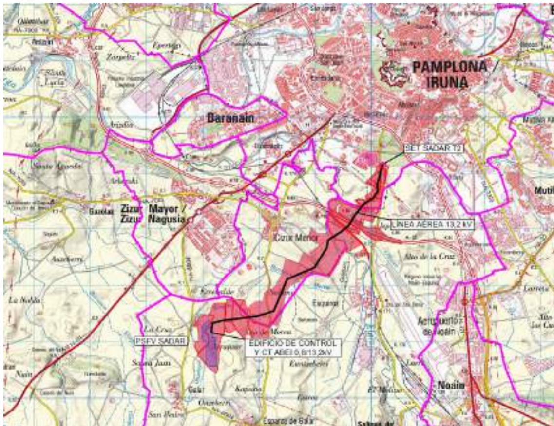
Imagen 1. Ubicación de la planta PSFV Sadar y su línea de evacuación.
