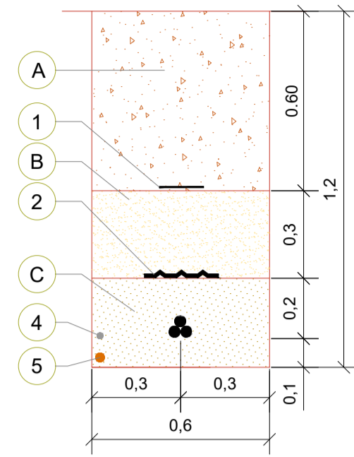
UNA TERNA (1T) - UN CIRCUITO (1C)
