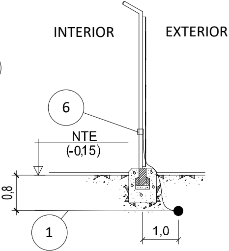
PUESTA A TIERRA DEL CERRAMIENTO
