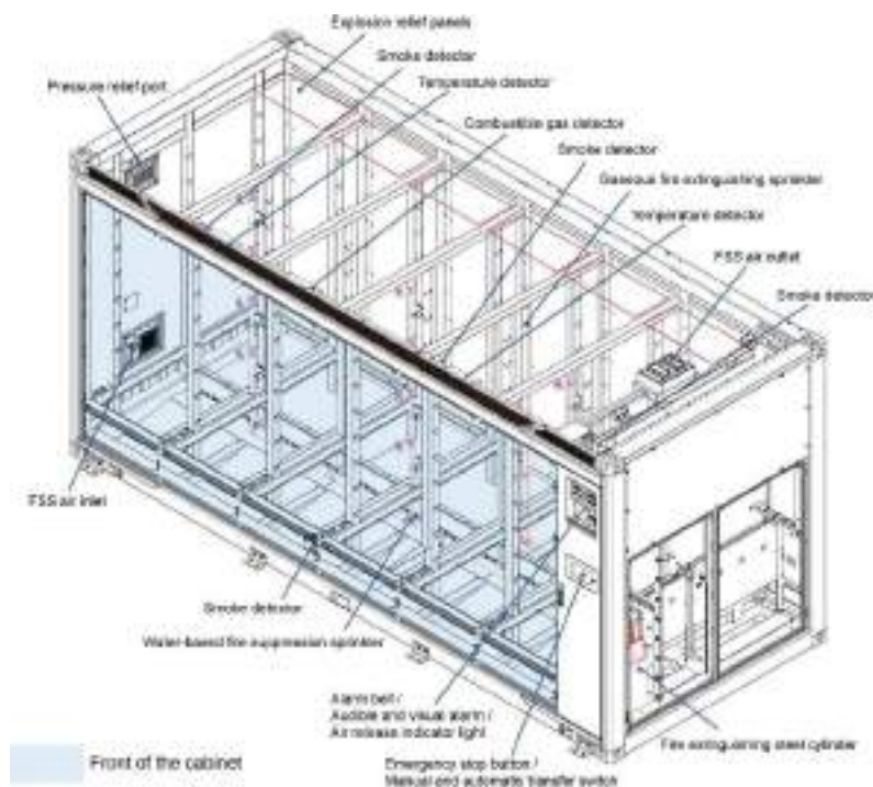
Figura 2 Disposición del SCI con FK5112
