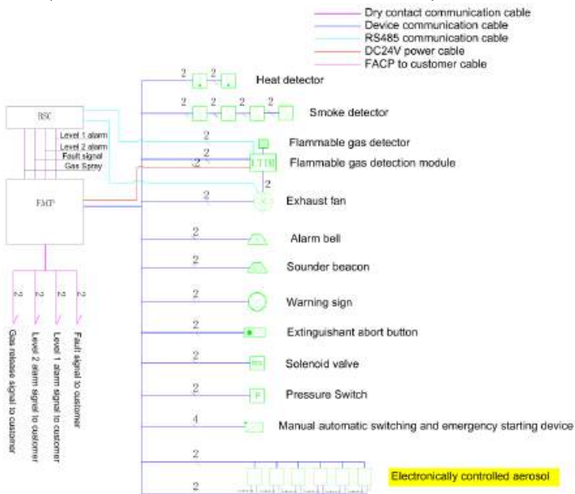
Figura 3 Esquema de comunicación del SCI
