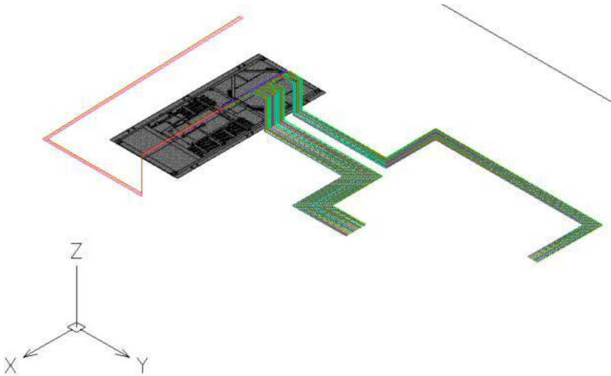
Figura 2. Conductores planteados para el cálculo del campo magnético
