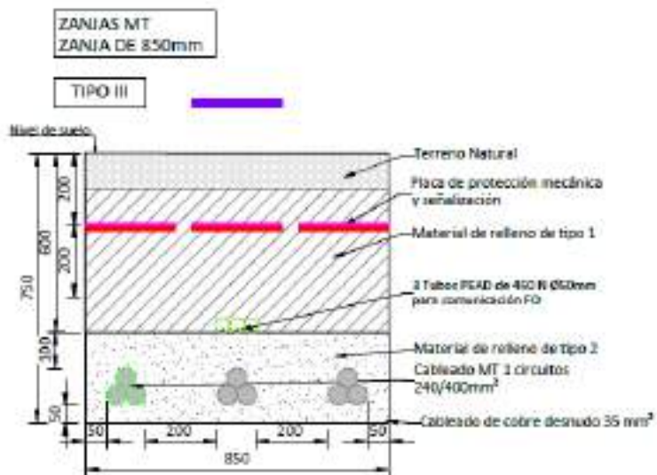
Figura 20 Detalle zanja MT III
