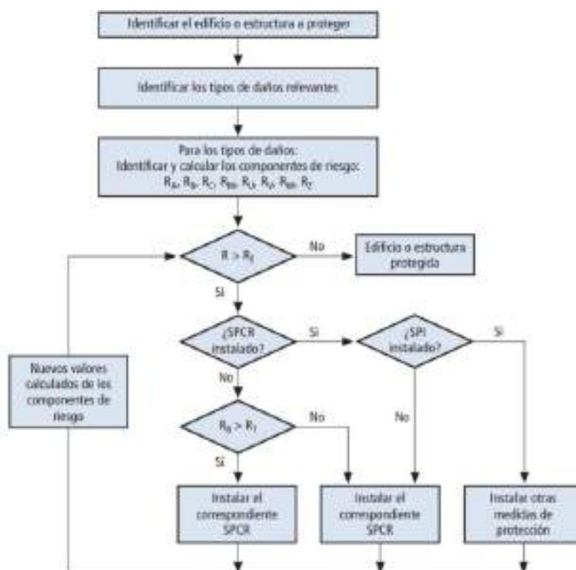
Figura 10 Diagrama de flujo para la elección de medidas de protección para los tipos de pérdida L1, L2 y L3
