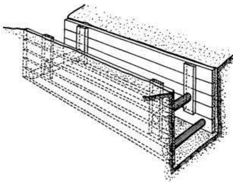
ENTIBACIÓN CUAJADA
