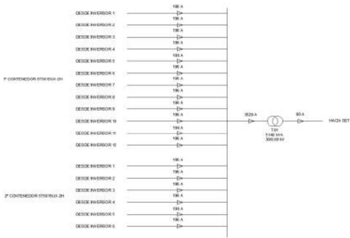
Figura 3. Esquema unifilar conductores
