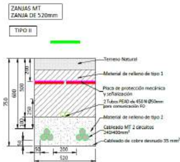
Figura 19 Detalle zanja MT II
