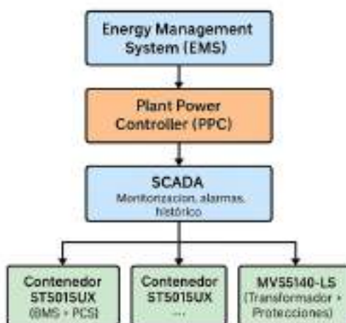
Figura 13 Esquema sistema de control simplificado
