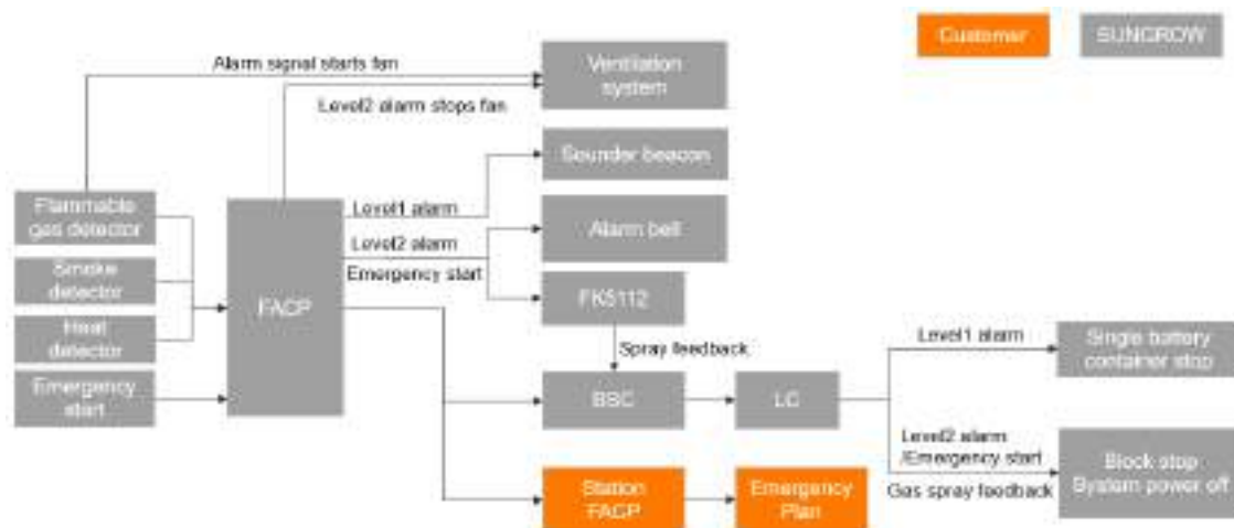
Figura 4 Lógica de control de la señal de incendio
