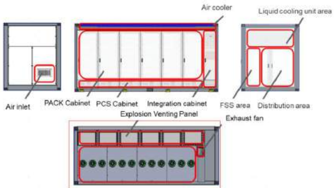
Figura 6 Layout del sistema de refrigeración
