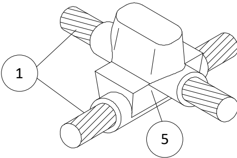
SOLDADURA ALUMINOTERMICA EN CRUZ
