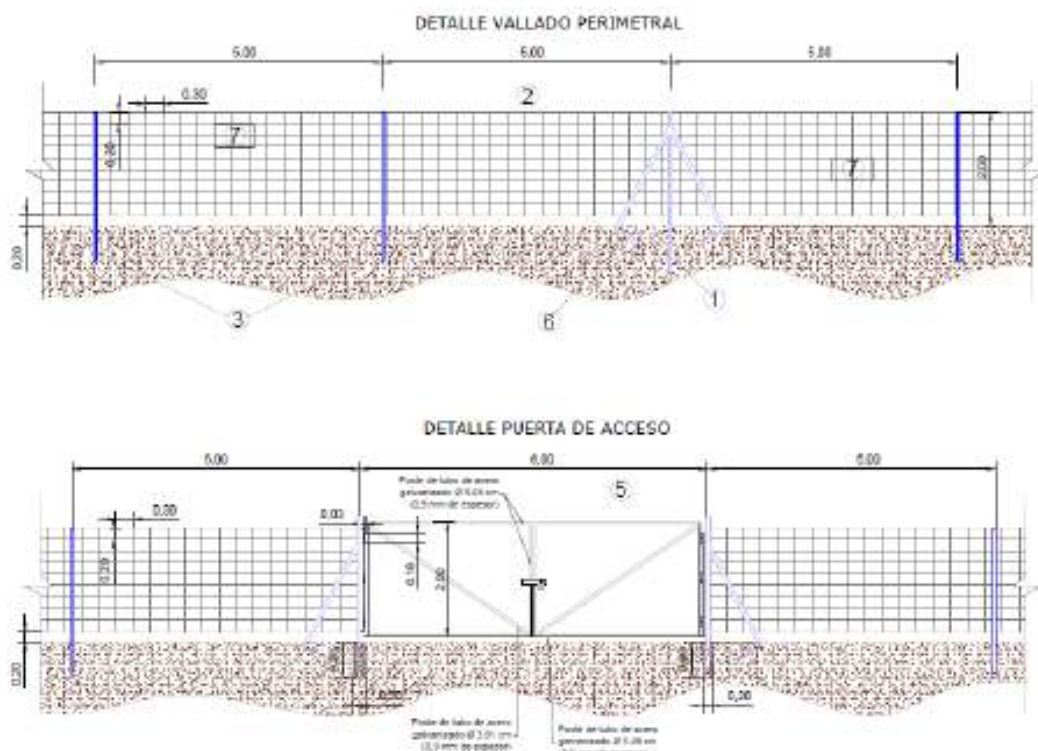
Figura 14 Detalle de vallado perimetral y la puerta de acceso
