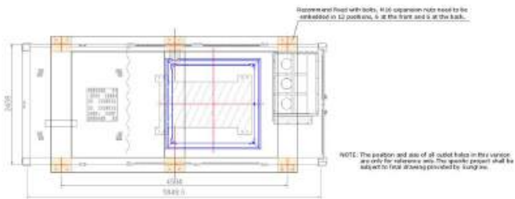
Figura 23 Detalle de cimentación de centro de transformación
