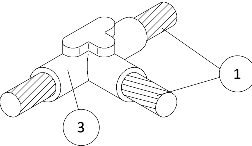
SOLDADURA ALUMINOTERMICA EN T CABLE Cu 150 mm2 A CABLE Cu 150 mm2
