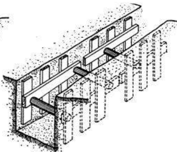
ENTIBACIÓN SEMICUAJADA
