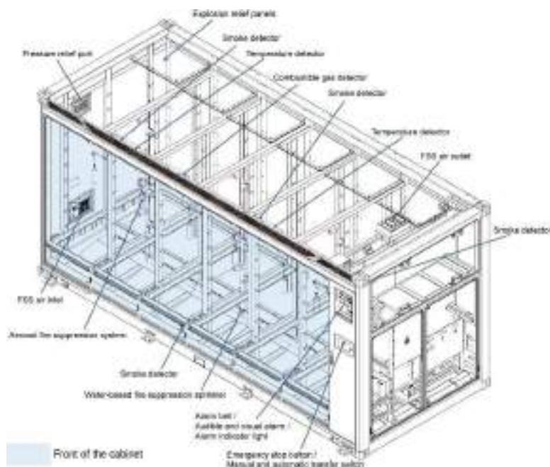
Figura 1 Disposición del SCI con Aerosol
