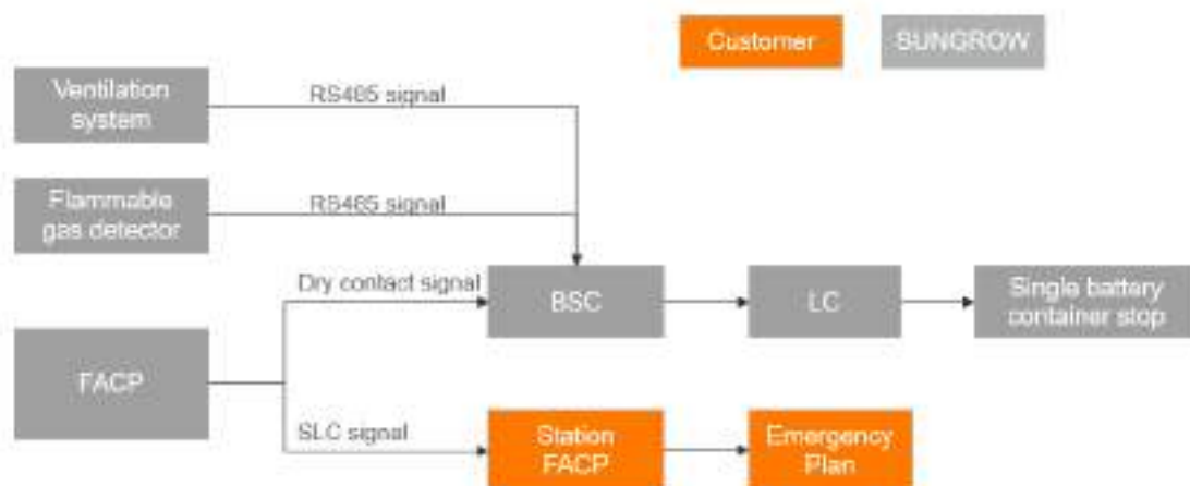
Figura 5 Lógica de control de la señal de falla
