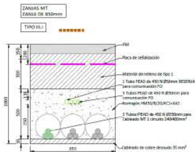
Figura 21 Detalle zanja MT I HM
