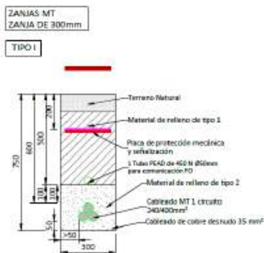
Figura 18 Detalles zanja MT I
