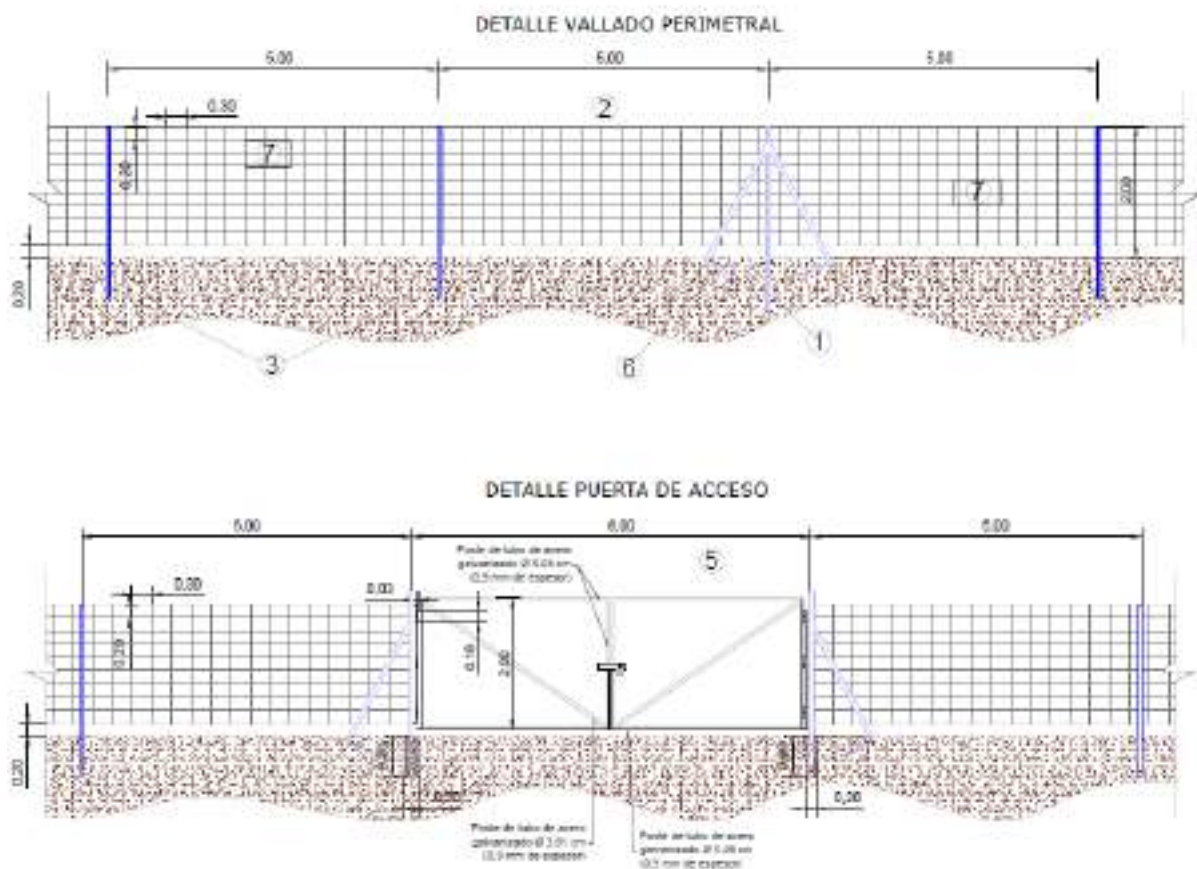
Figura 7 Detalle de vallado perimetral y la puerta de acceso
