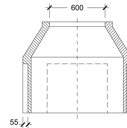
SECCIÓN DE ALZADO A-A'
