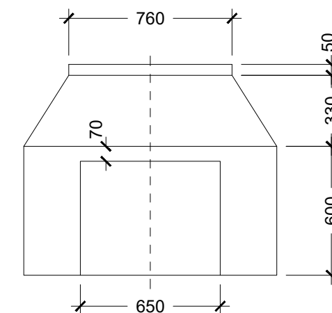
VISTA DE ALZADO
