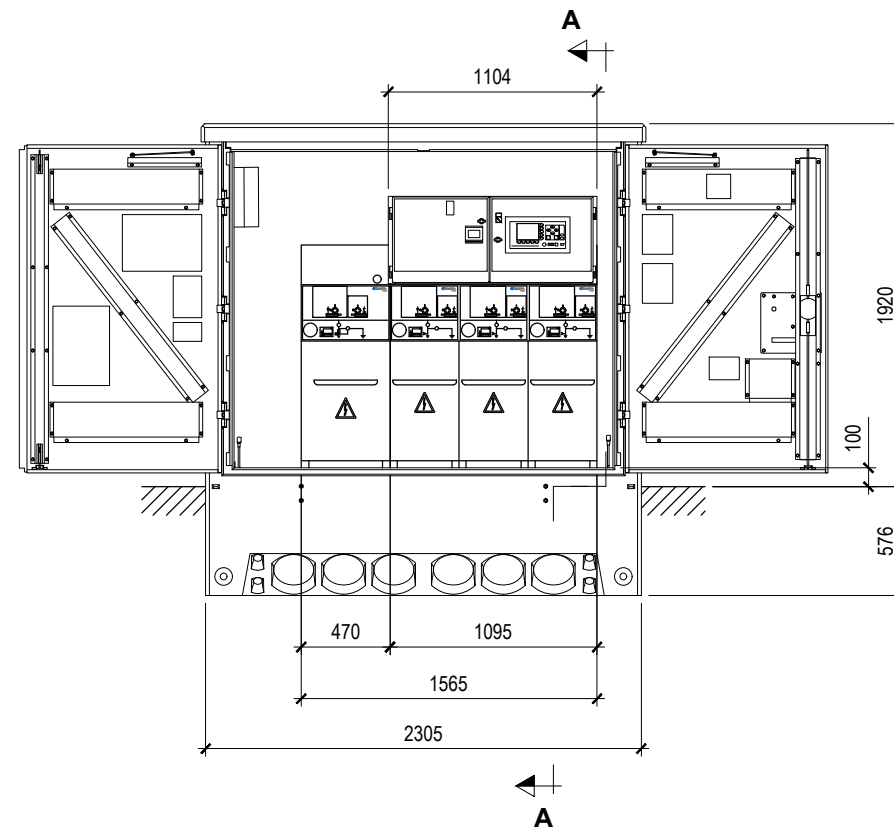
VISTA FRONTAL PUERTAS ABIERTAS
