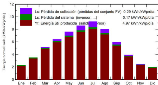
Producciones normalizadas (por kWp instalado)
