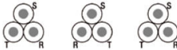
Figura 22: Colocación de cables en tresbolillo.
