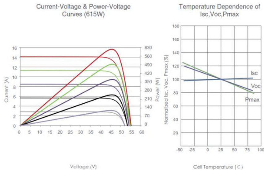
Figura 20: Curvas Características JKM625N-78HL4.
