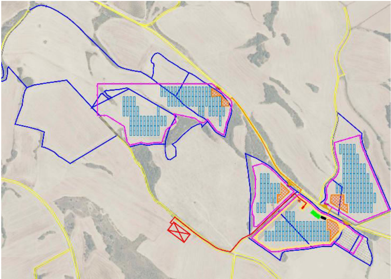
Figura 18: Instalación FV.
