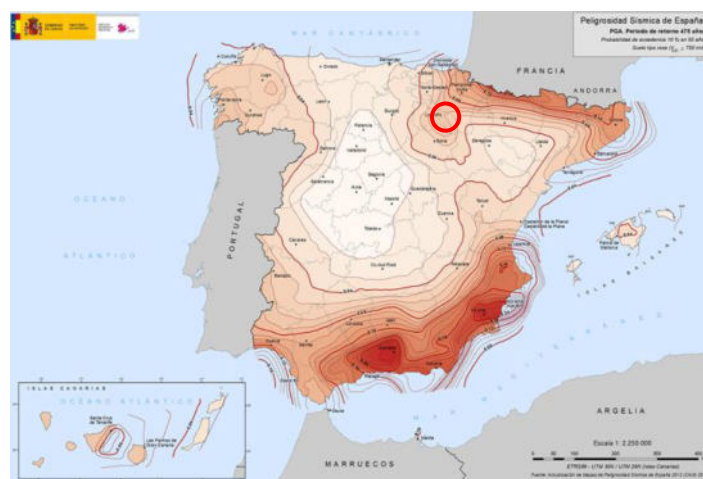
Figura 9: Mapa Riesgo sísmico.
