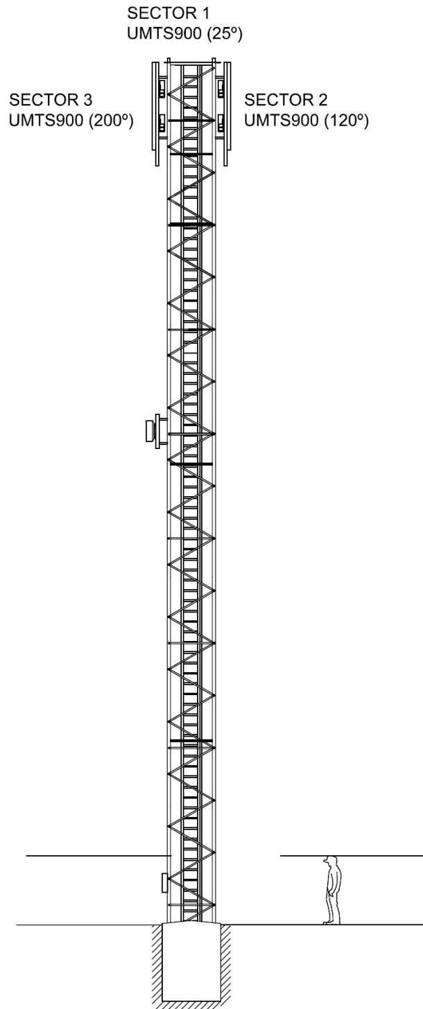
Plano de instalación (alzado).
