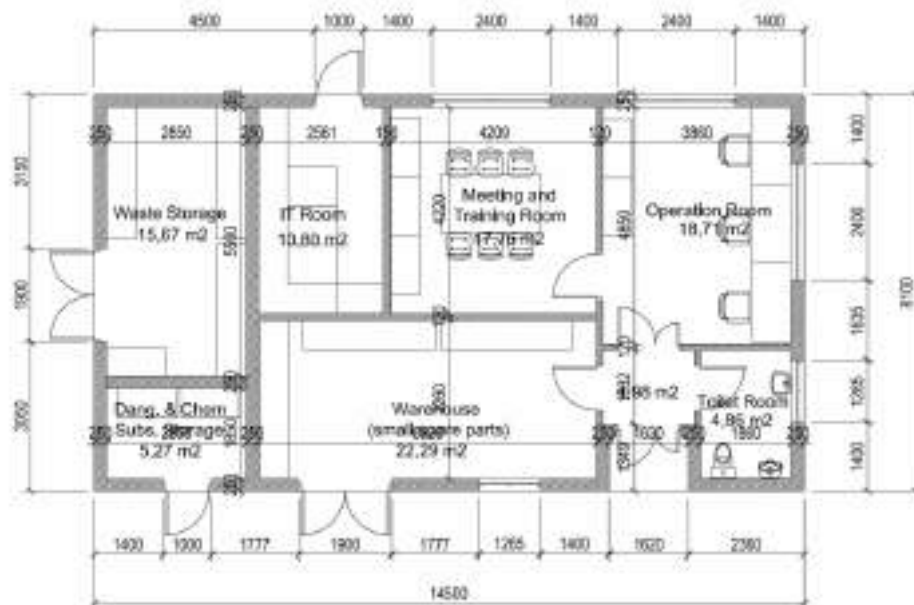
Imagen 4. Planta tipo del edificio O&M
