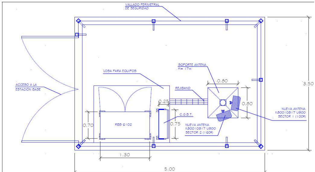
Plano de instalación (planta).
